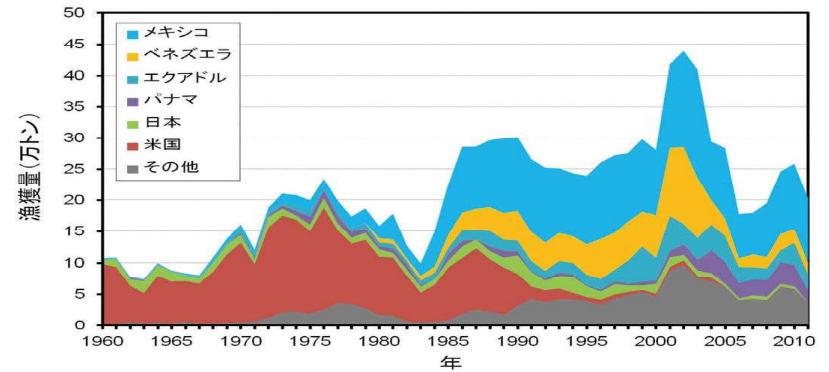
東部太平洋
