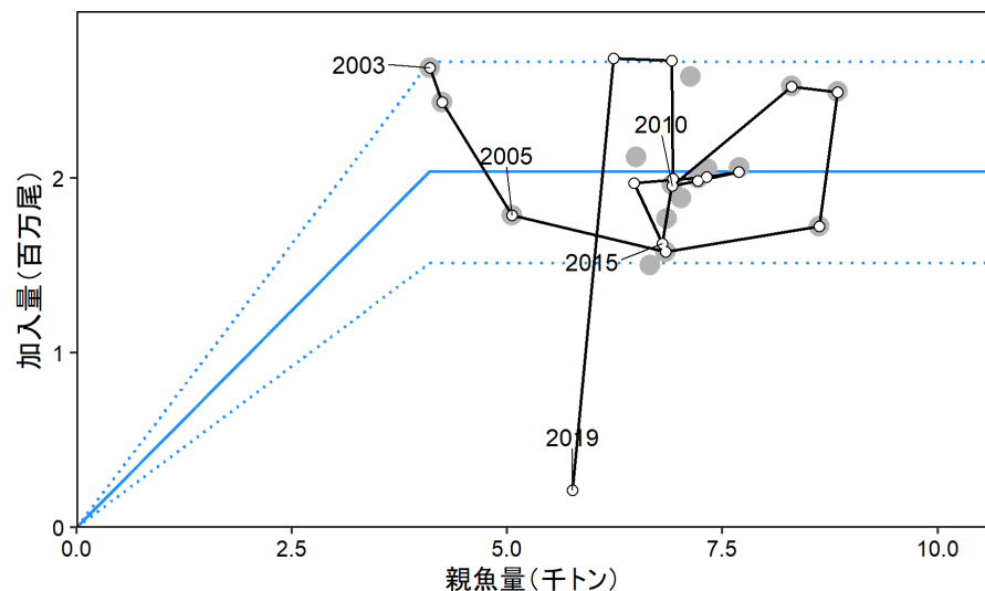
図4 再生産関係
