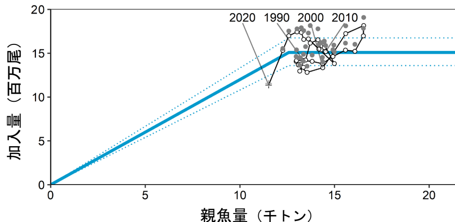
図4 再生産関係
