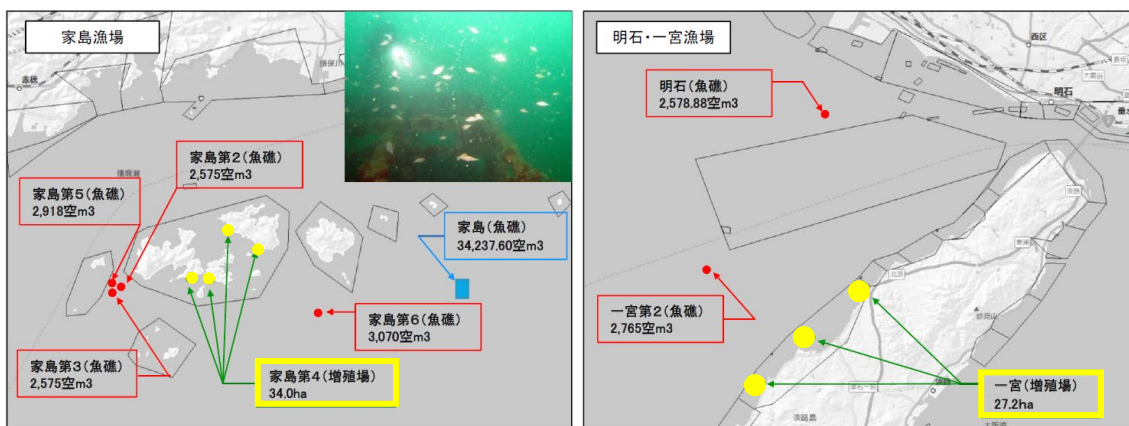
水産環境整備事業 A地区 事業概要図(便益算定対象施設を黄で着色)
