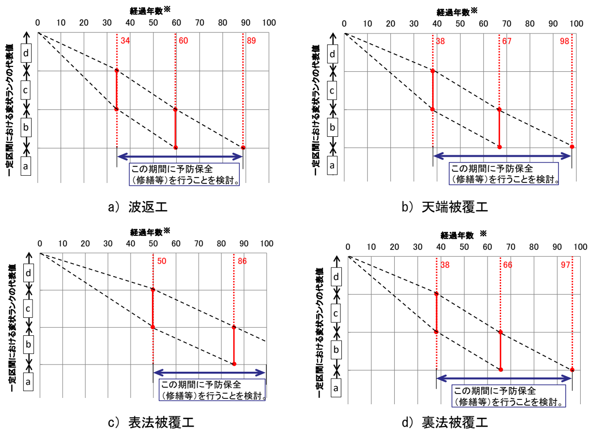
図-7.8 護岸の場合の部位・部材ごとの劣化予測と修繕等の時期
