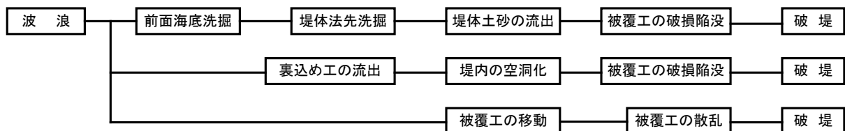
図-5.12 緩傾斜護岸の変状連鎖
