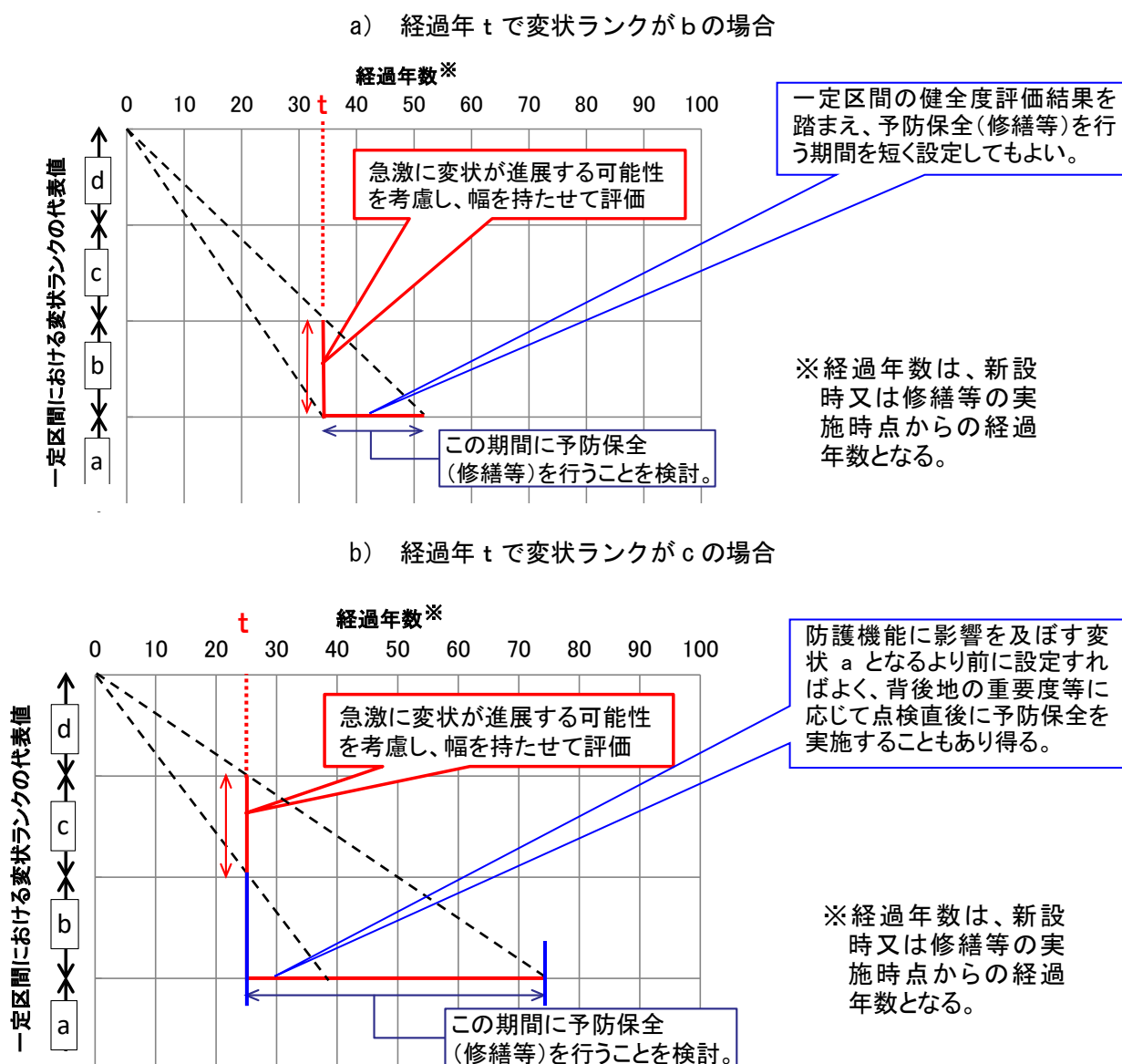
図-7.6 劣化予測と修繕時期のイメージ
