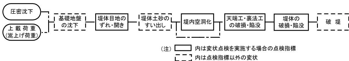
図-5.11 護岸・堤防の変状連鎖
