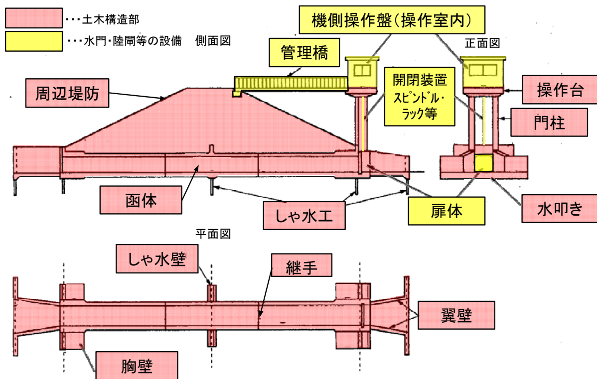
図-2.8 樋門・樋管の点検位置
