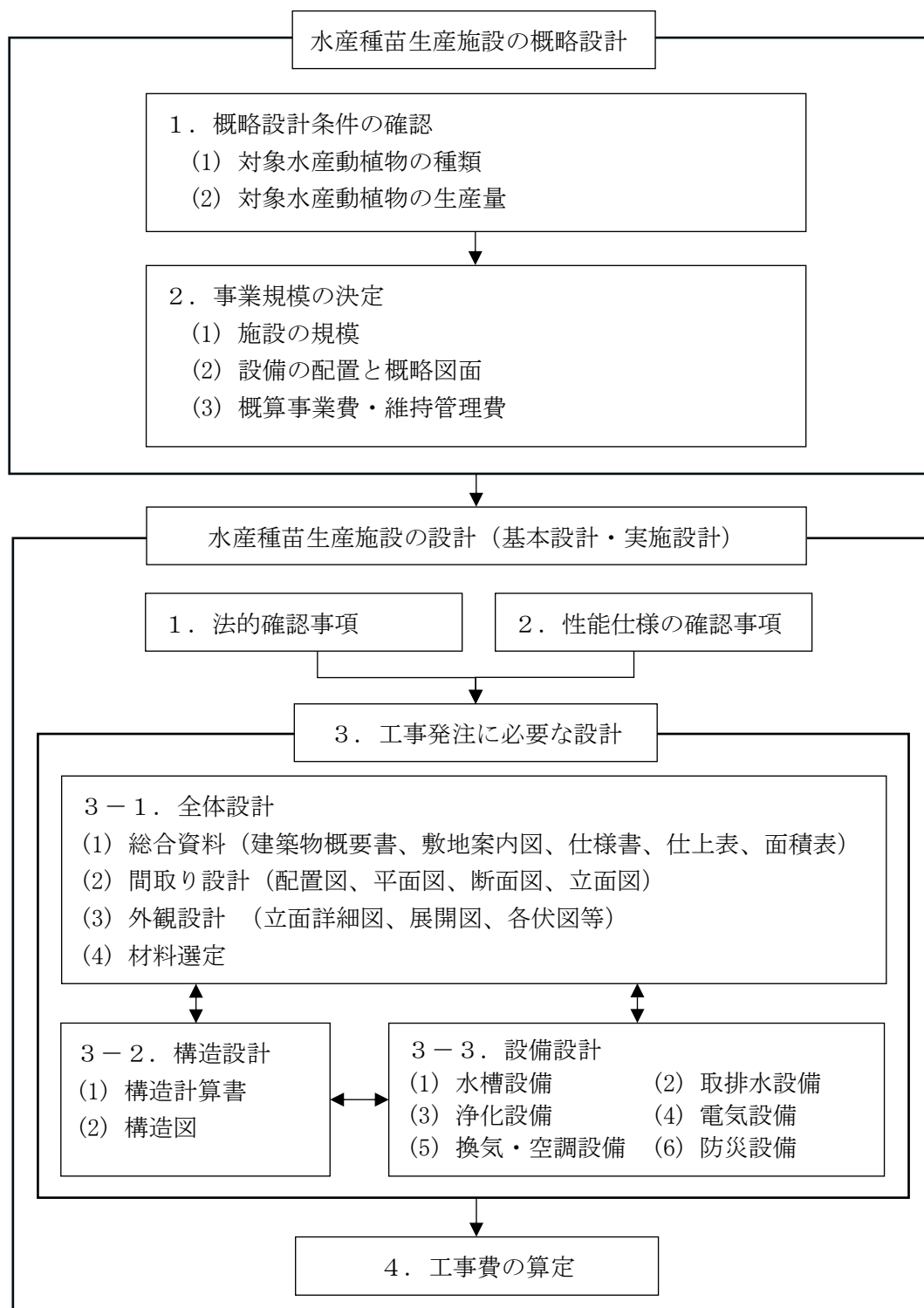
図-10-1-1 水産種苗生産施設の設計フロー
