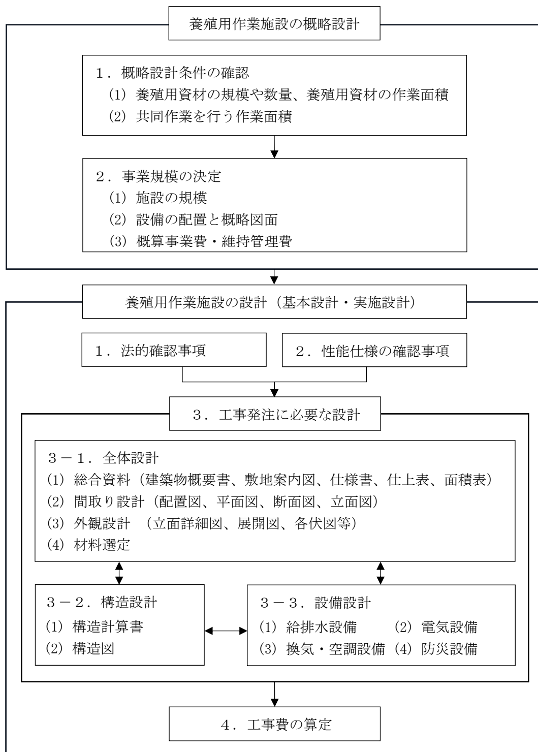
図-12-1-1 養殖用作業施設の設計フロー
