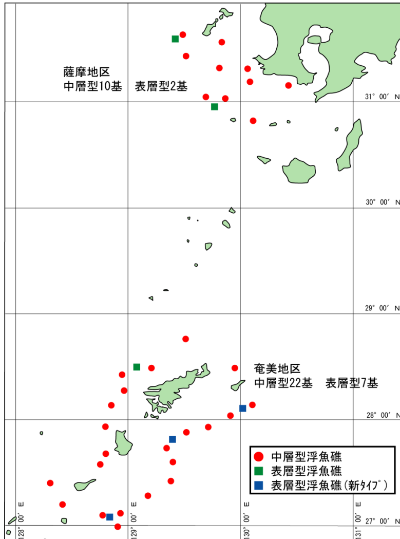
図 31 鹿児島県沖の浮魚礁の設置位置
