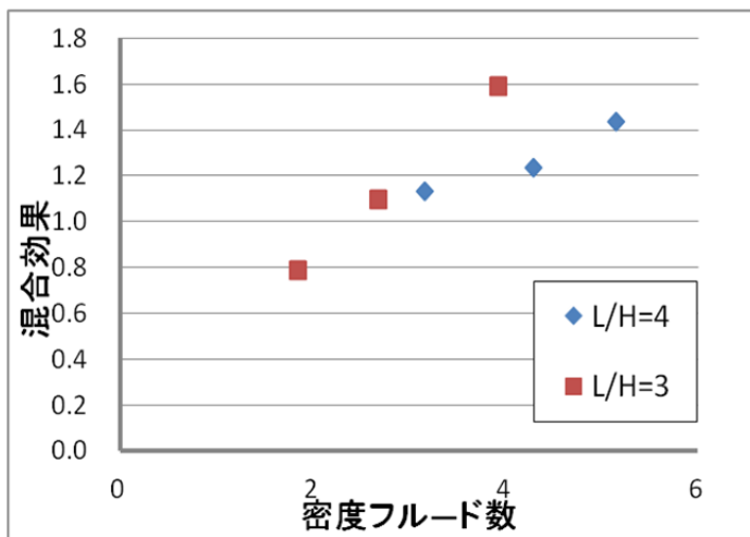
図-3 密度フルード数と混合効果の関係
