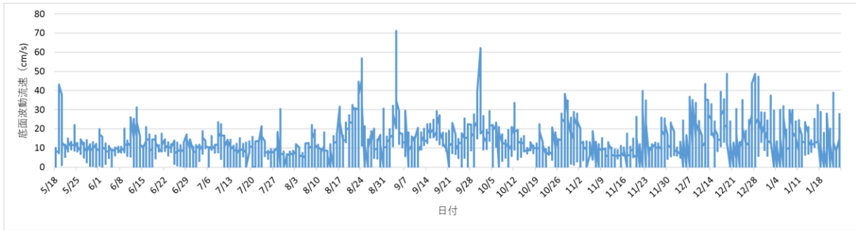
図 3.2.2.2-1 平成 30 年度小鈴谷試験区における底面波浪流速値の推移
