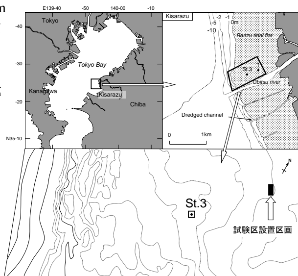
図 1.2.3.1-1 調査地の概要（久津間地区）
