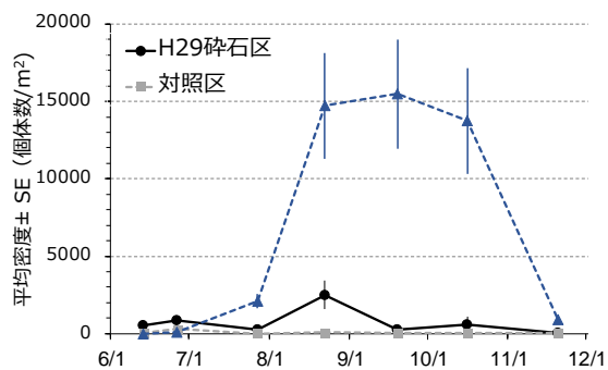
図 3.2.3.2-1 船橋地区試験区におけるホトトギスガイ個体密度
