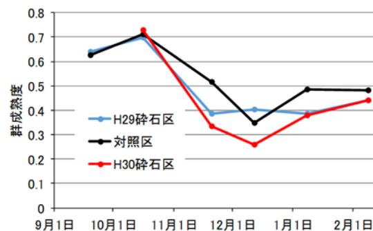
図 1.2.3.2-10 船橋地区産アサリの群成熟度
