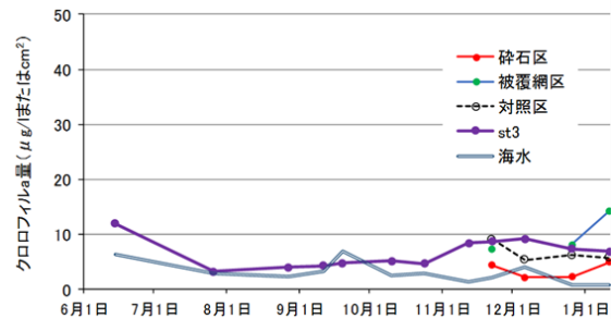
図 1.2.3.2-5 久津間地区のクロロフィル a 量および濃度
