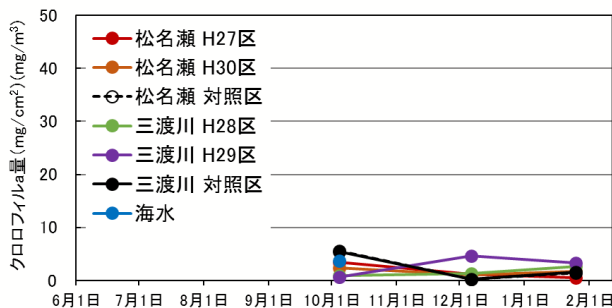
図 1.2.1.2-1 三重県松阪地区のクロロフィル a 量
