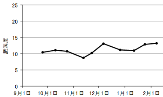
図 1.2.3.2-7 久津間地区産アサリの肥満度
