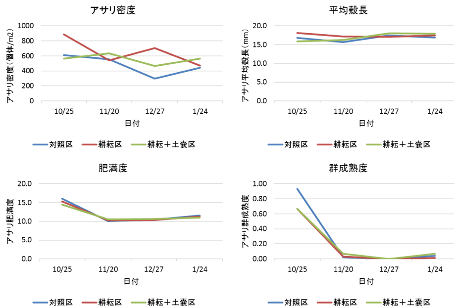
図 3.2.2.2-3 各試験区のアサリ密度、平均殻長、平均肥満度、群成熟度の推移
