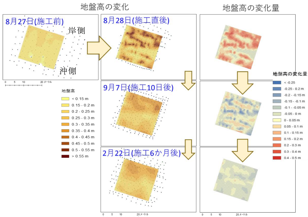
図 2.2.3.2-1 施工前および施工後における地盤高の変化および変化量の推移
