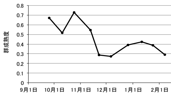
図 1.2.3.2-8 久津間産アサリの群成熟度
