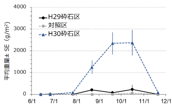
図 3.2.3.2-2 船橋地区試験区におけるホトトギスガイ重量密度
