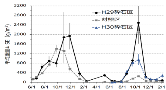
図 1.2.3.2-4 船橋地区試験区におけるアサリ重量
