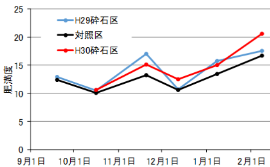
図 1.2.3.2-9 船橋地区産アサリの肥満度
