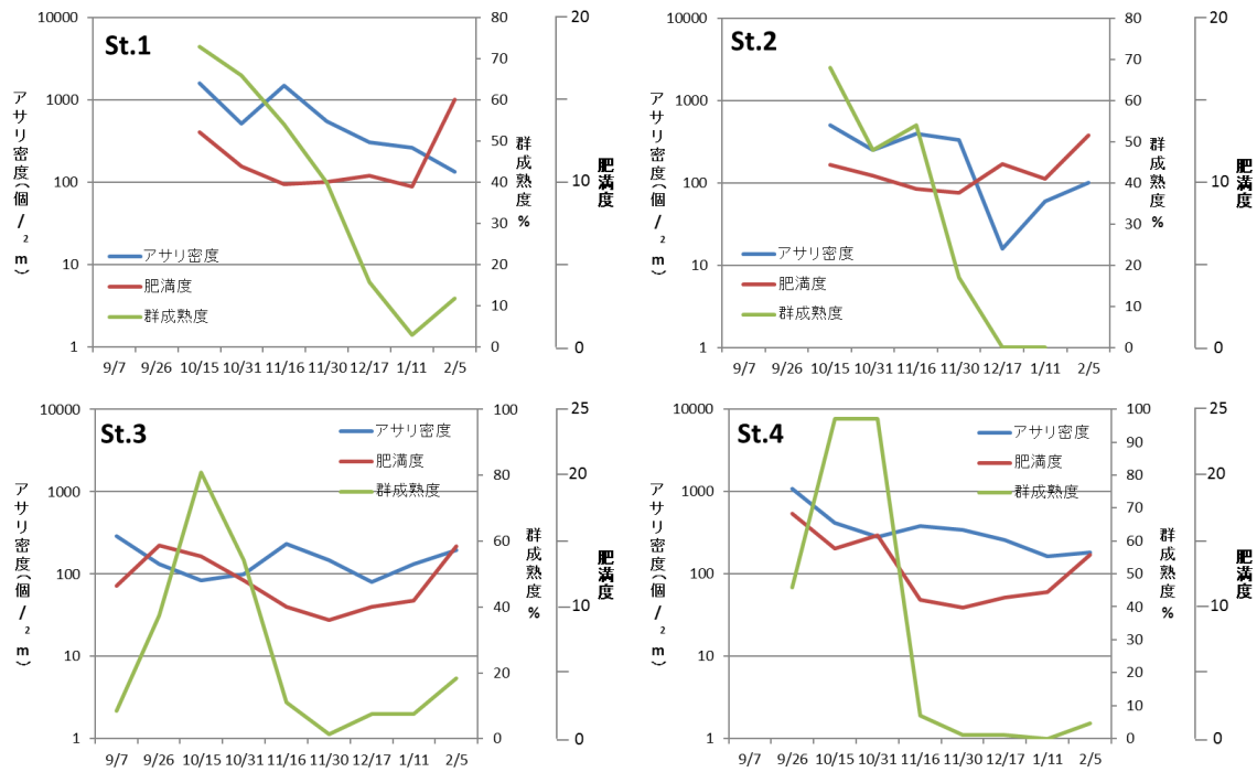
図 1.2.2.2-2 各定点のアサリ密度、肥満度、群成熟度の推移
