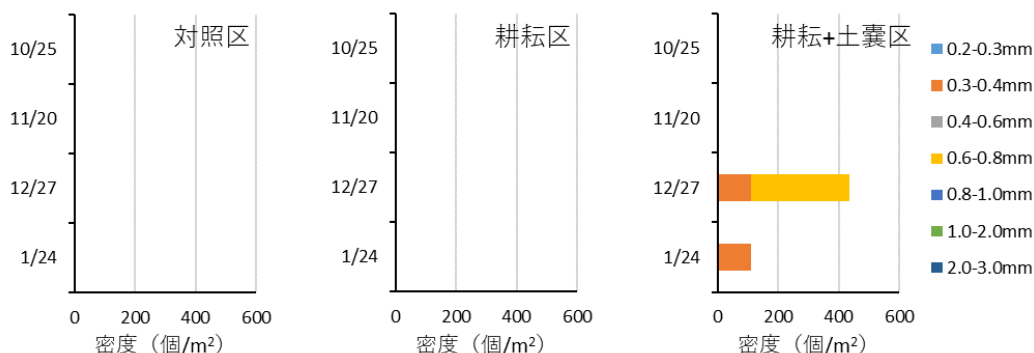
図 3.2.2.2-4 各試験区における着底稚貝、初期稚貝密度の推移
