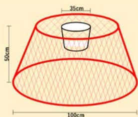
カゴトラップの模式図
