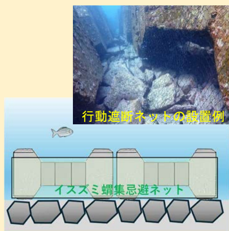
図 H-5 イスズミ蛸集忌避対策のイメージ
