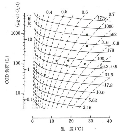
図 6.2 砂浜のCOD除去機能に関するCOD負荷(L)-温度ダイアグラム
