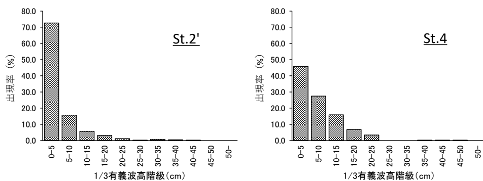
図 9 有義波高階級別出現頻度 (夏季)
