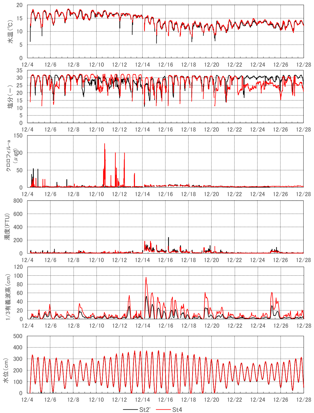
図 10 連続観測結果 (冬季)
