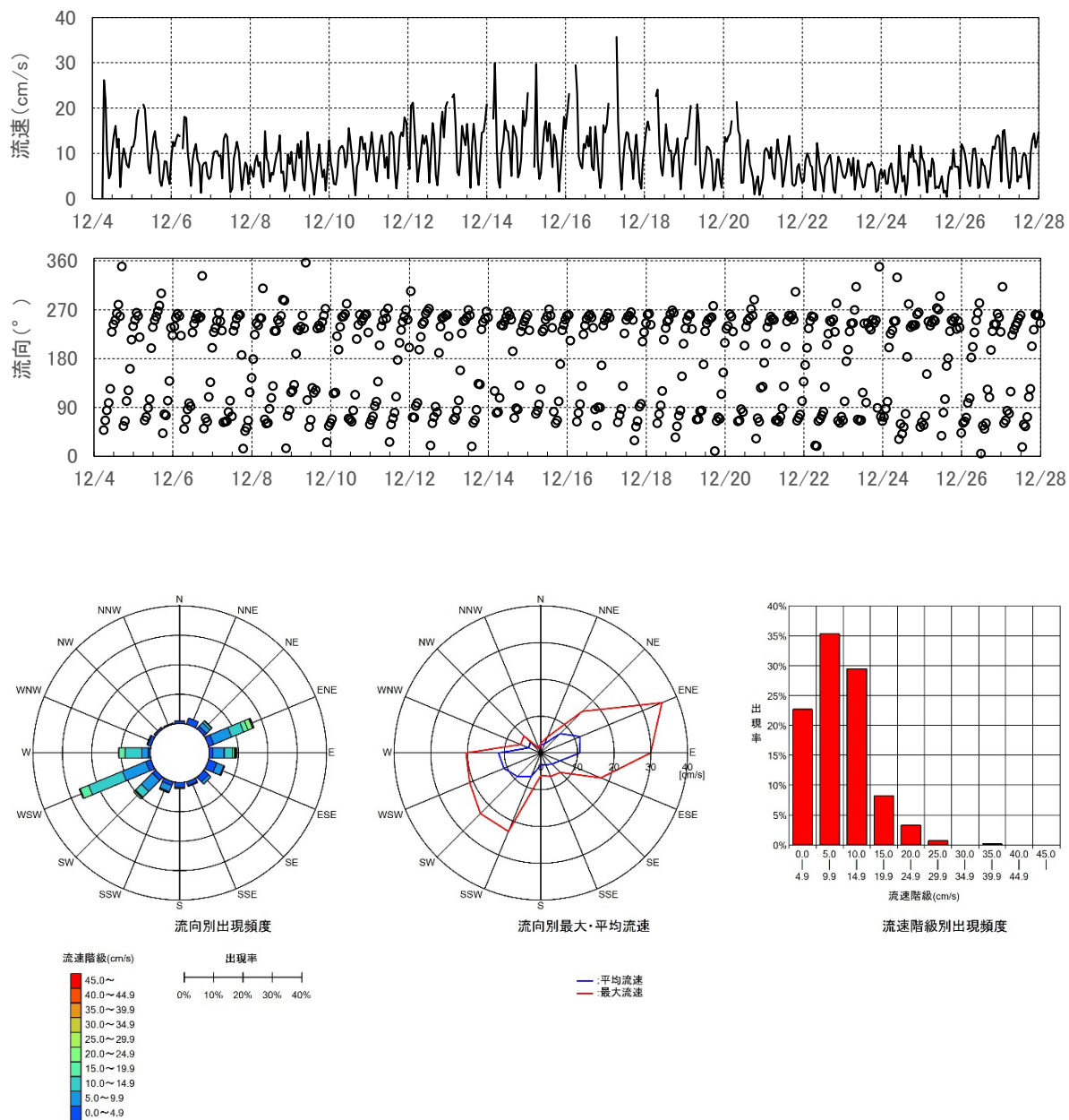
図 11 流況連続観測結果 (St. 2' 冬季)
