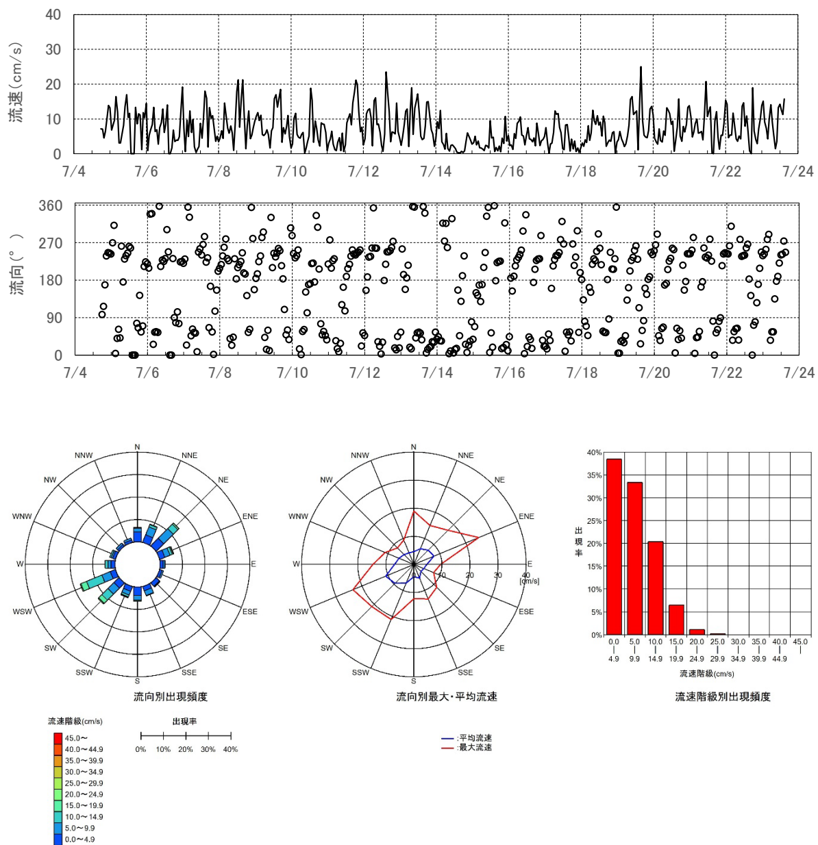
図 7 流況連続観測結果 (St. 2' 夏季)
