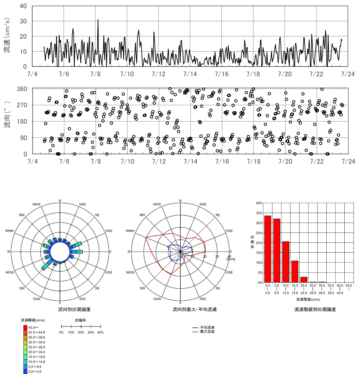
図 8 流況連続観測結果 (St. 4 夏季)
