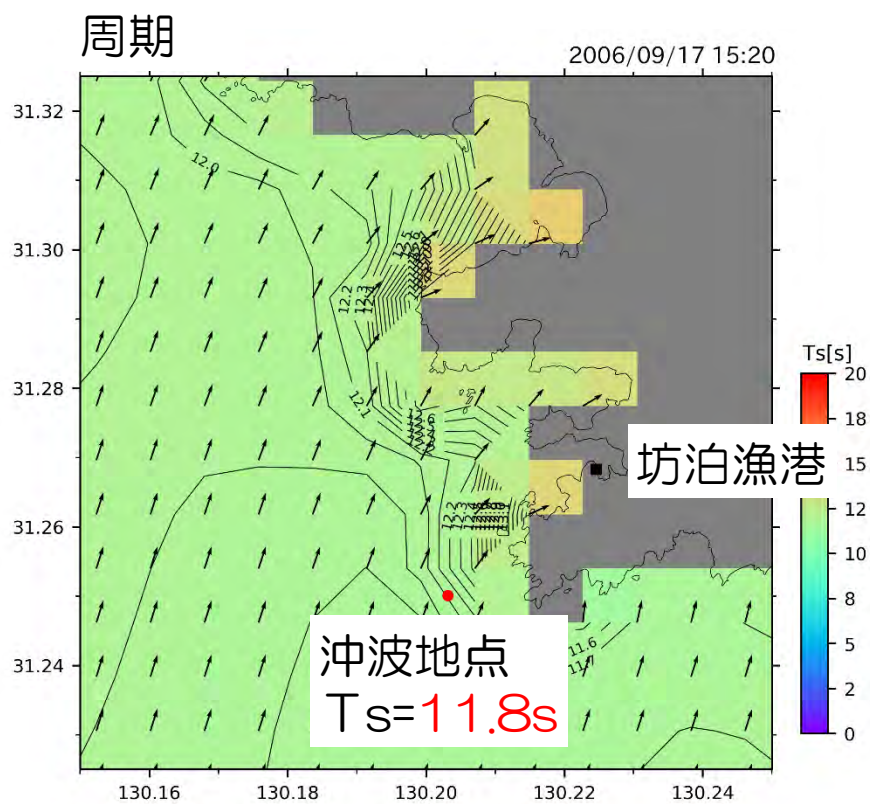
図 4-11(2) 推算周期・波向の平面分布 (2006年9月17日15:20)
