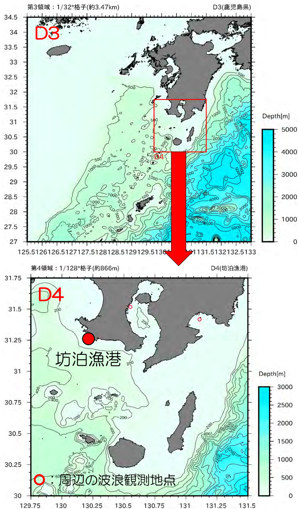
図 4-10 (2) 波浪推算の計算領域 (上段 : 第3領域、下段 : 第4領域) (第3領域 : 1/32°格子 (約3.47km) 、第4領域 : 1/128°格子 (約0.86km) )
