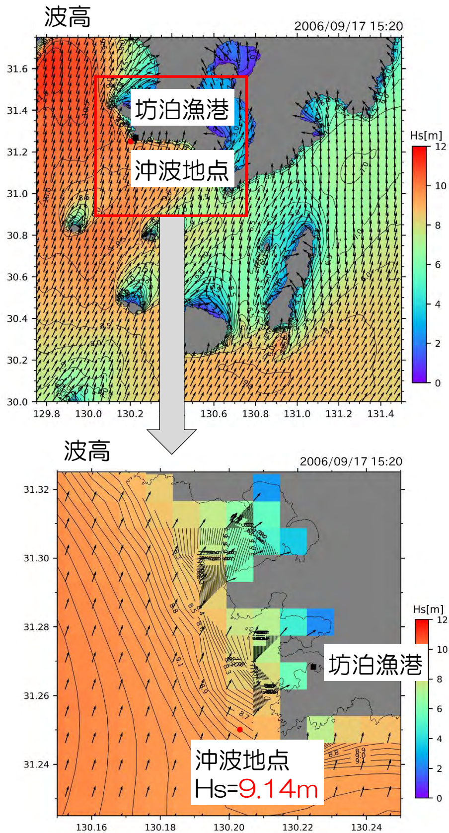
図 4-11(1) 推算波高・波向の平面分布 (2006年9月17日15:20)
