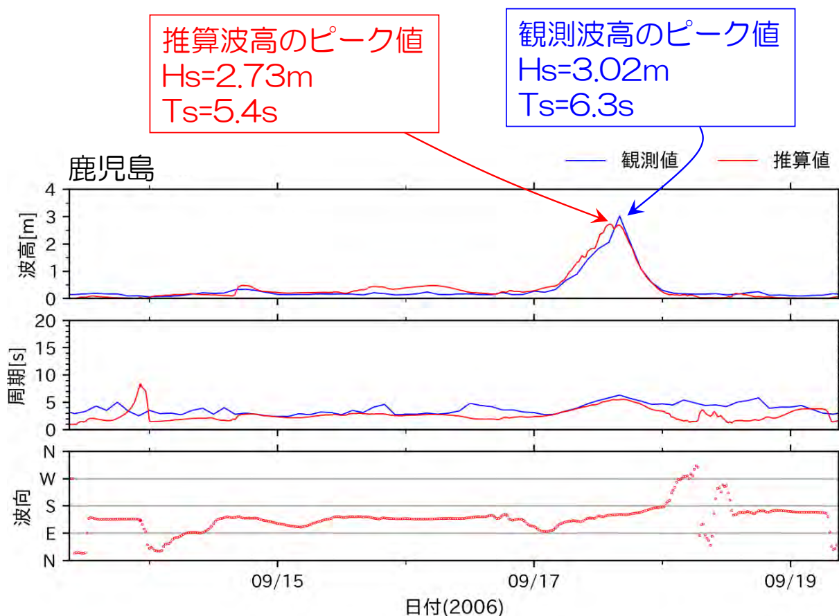
図 4-12 波浪推算結果と観測結果の比較
