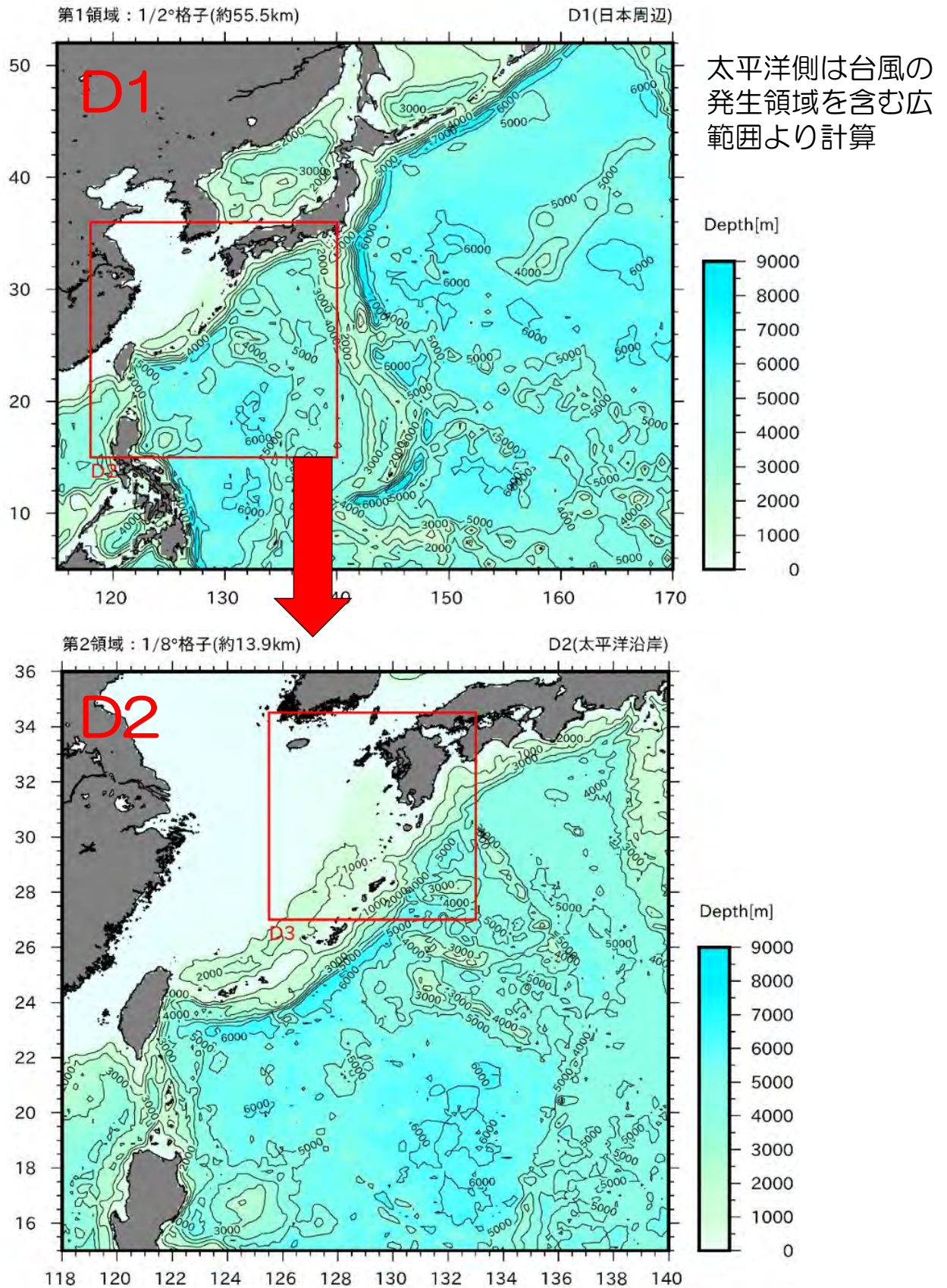
図 4-10 (1) 波波浪推算の計算領域（上段：第1領域、下段：第2領域） （第1領域：1/2°格子（約55.5km）、第2領域：1/8°格子（約13.9km））
