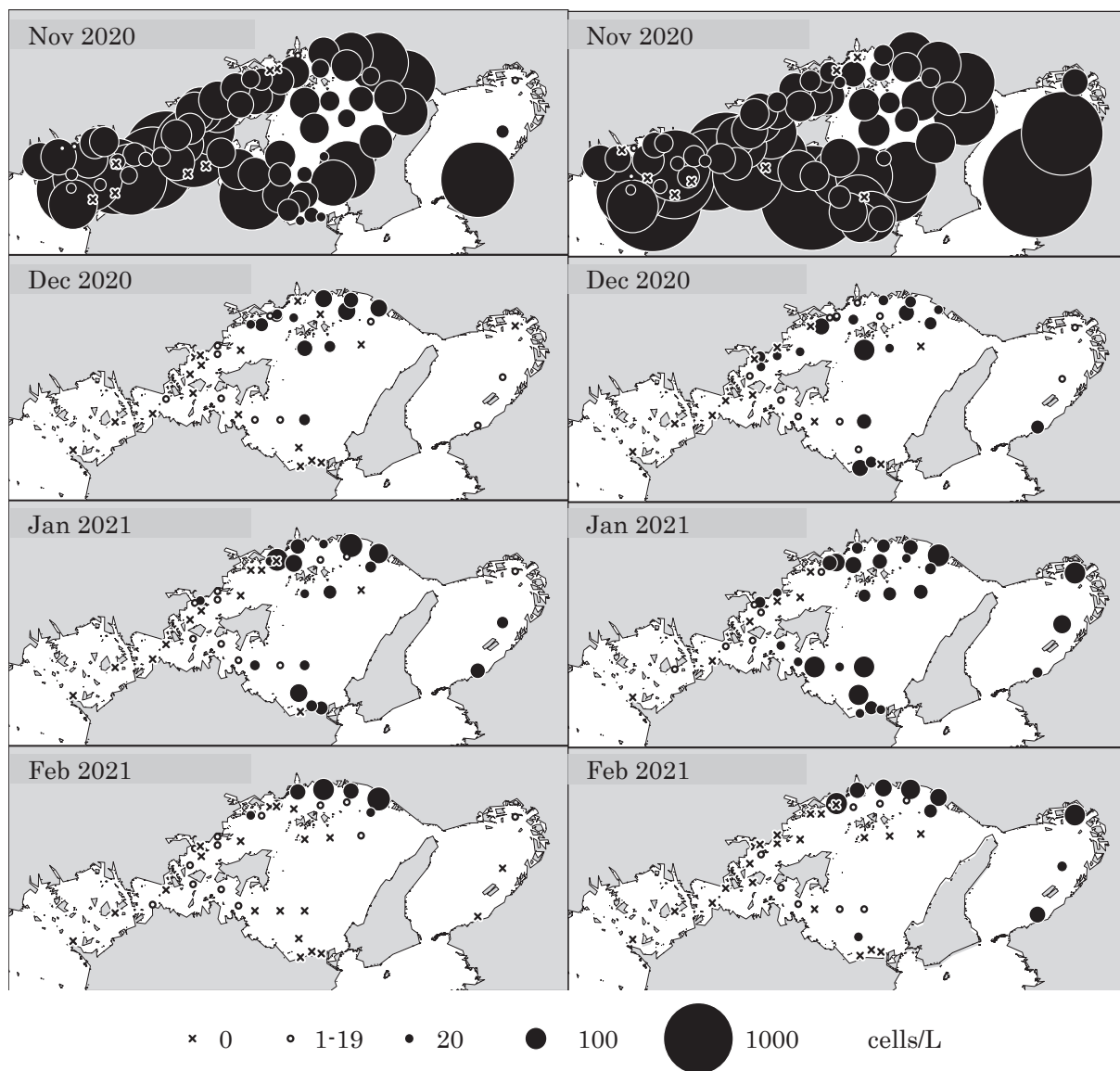
図 44 2020 年漁期における Coscinodiscus wailesii 細胞密度の水平分布（単位：cells/L）
