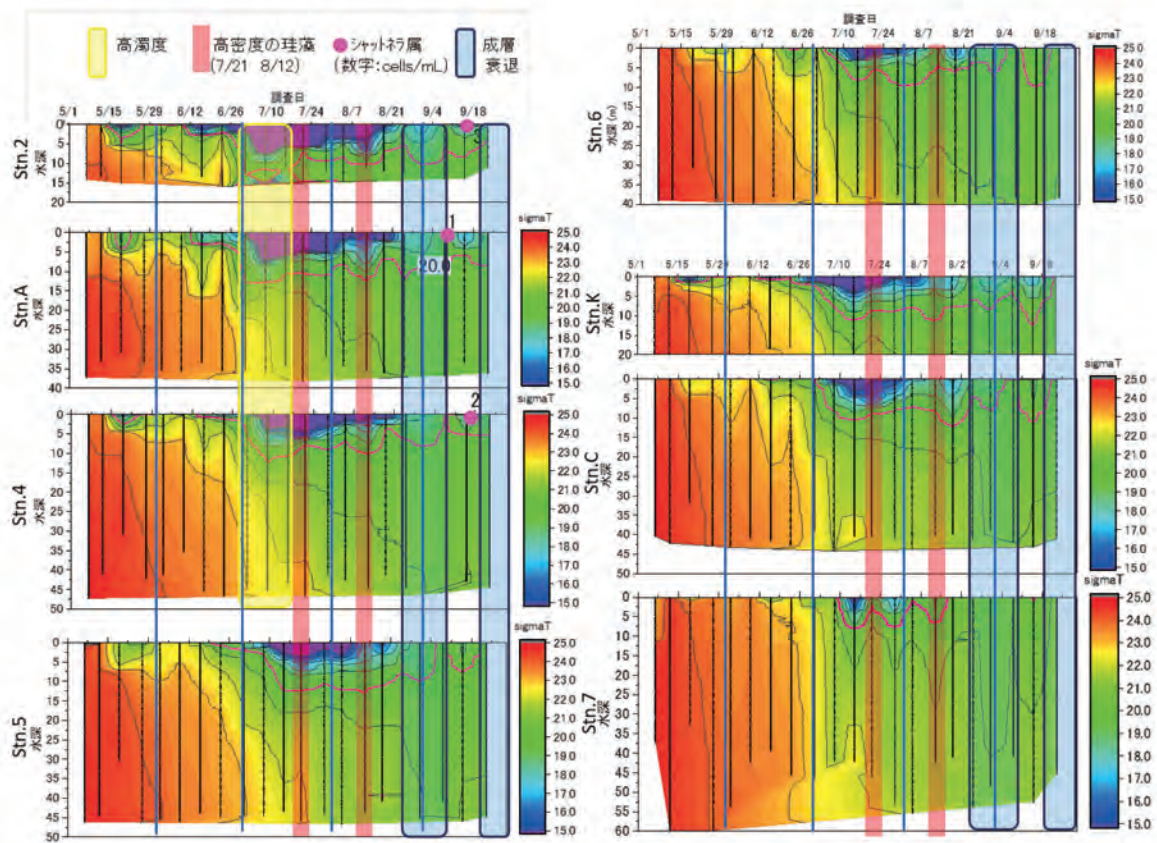
図 13. 八代海 8 定点における Sigma-T の推移 (ピンク線 : 20).
