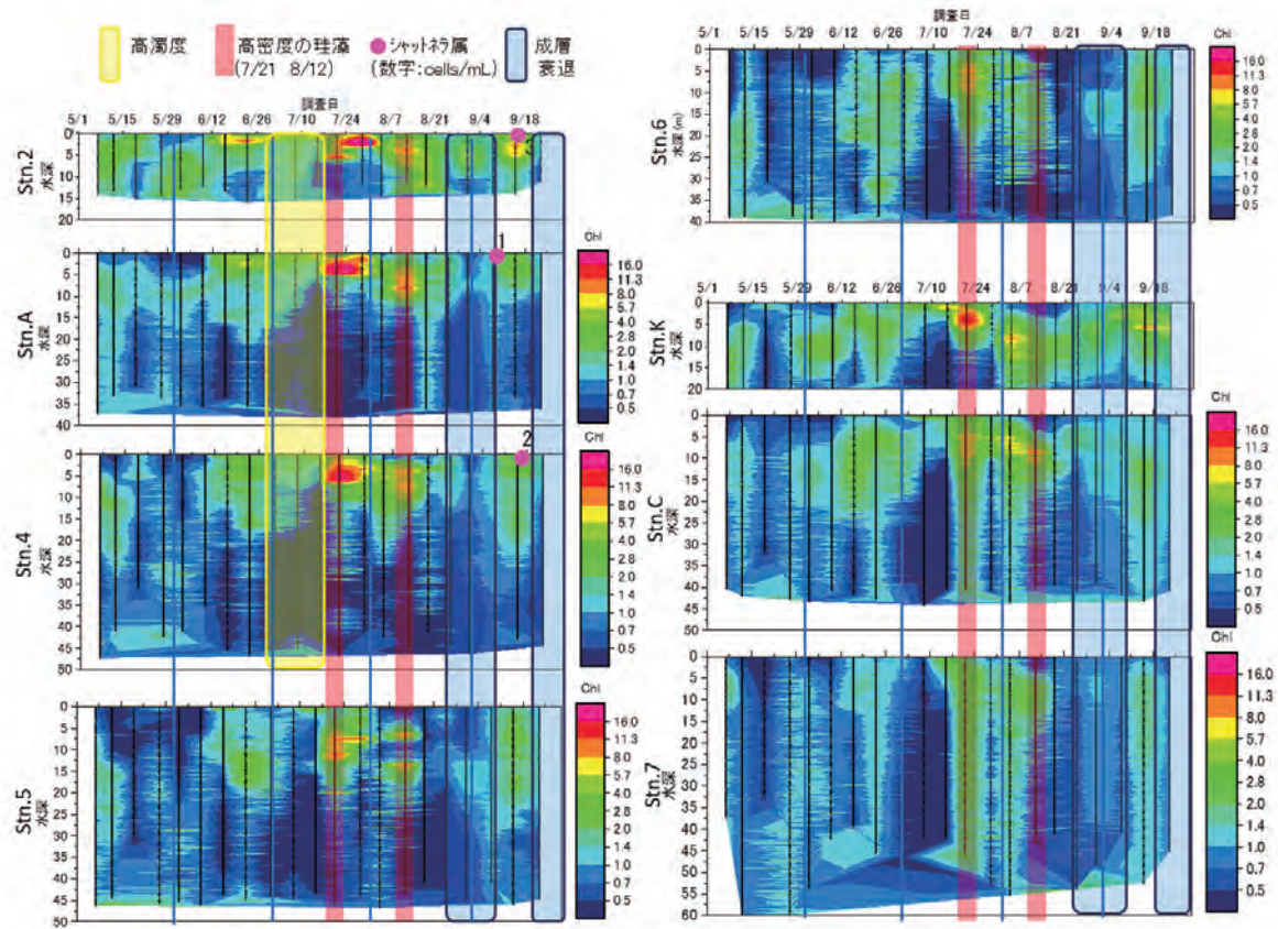
図 14. 八代海 8 定点におけるクロロフィル蛍光値の推移.
