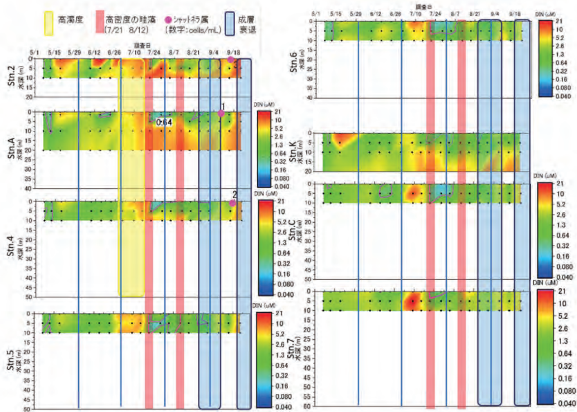
図 15. 八代海 8 定点における DIN 濃度の推移 (ピンク線：半飽和定数 0.65 \mu\text{M} ).
