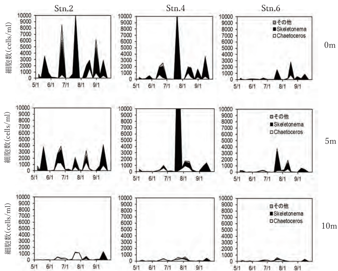
図 18-1. 八代海 (Stn. 1~6) における珪藻類の推移.
