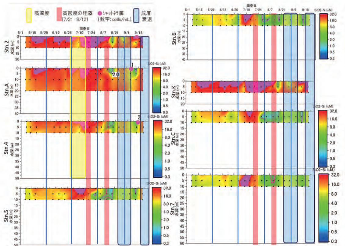
図 16. 八代海 8 定点における DIP 濃度の推移 (ピンク線：半飽和定数 0.25 \mu\text{M} ).
