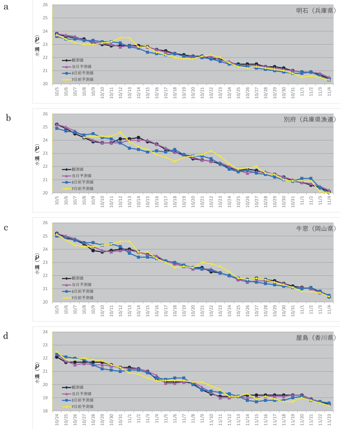
図 6. 水温の観測値と当日、3 日前及び 7 日前予報値との比較（令和 2 年 10～11 月） a. 明石（兵庫県）、b. 別府（兵庫県漁連）、c. 牛窓（岡山県）、d. 屋島（香川県）
