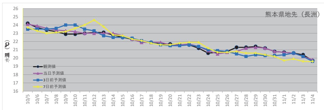
図7. 水温の観測値と当日、3日前、及び7日前予報値との比較（令和2年10～11月）
