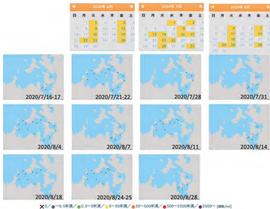
図2.「赤潮分布情報」で収集・公表された伊万里湾における有害赤潮原因種カレンニア ミキモトイの細胞密度の分布（長崎県水産試験場、佐賀県玄海水産振興センターの調査結果による。カレンダーの黄色表示は、公表データが有ることを示す。）
