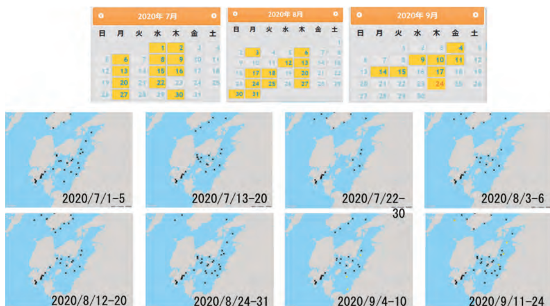
図 4.「赤潮分布情報」で収集・公表された八代海における有害赤潮原因種シャットネラ属の細胞密度の分布（熊本県水産研究センター，鹿児島県水産技術開発センター，天草市水産研究センター，熊本県海水養殖漁業協同組合，東町漁業協同組合，水産研究・教育機構の調査結果による。カレンダーの黄色表示は，公表データが有ることを示す。）
