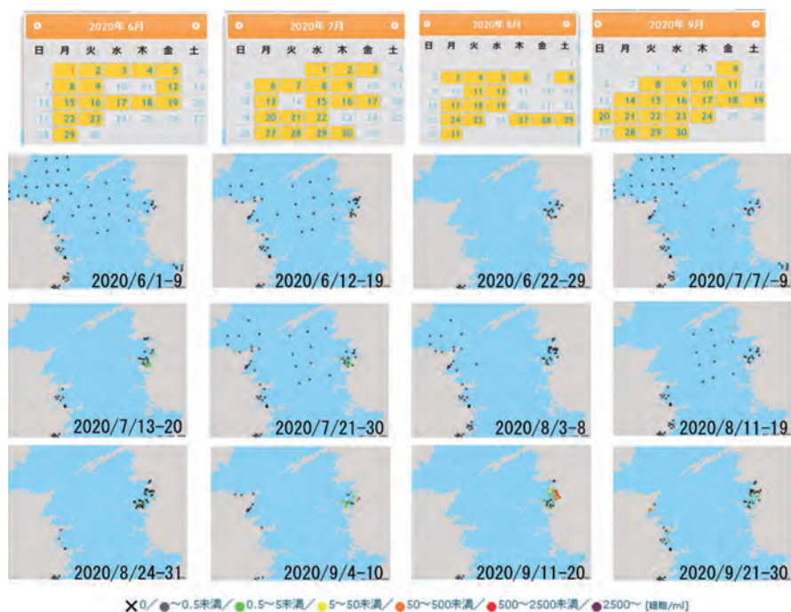
図3.「赤潮分布情報」で収集・公表された豊後水道における有害赤潮原因種カレンニア ミキモトイの細胞密度の分布（大分県農林水産研究指導センター水産研究部、愛媛県農林水産研究所水産研究センター他の調査結果による。カレンダーの黄色表示は、公表データが有ることを示す。）
