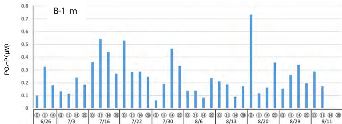
図 2-1-4. 調査点ごとの栄養塩濃度 (PO 4 -P)
