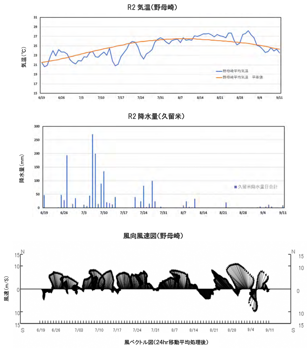
図 2-1-2. 調査期間中の気温、降水量及び風向風速
