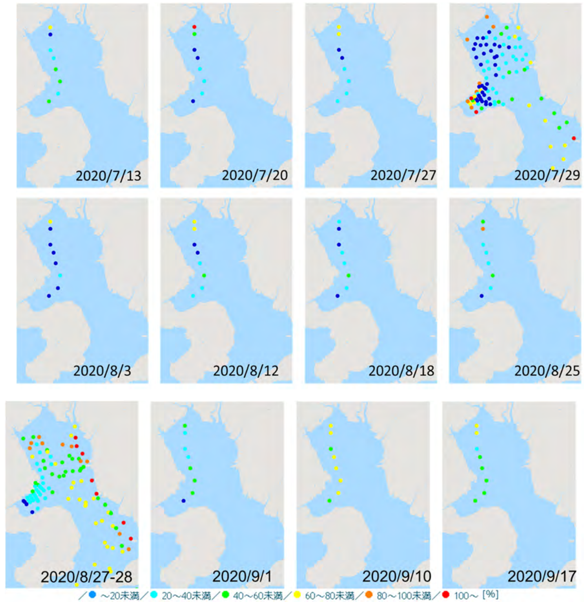
図 1-2-15. 有明海の底層の溶存酸素(%)の分布
