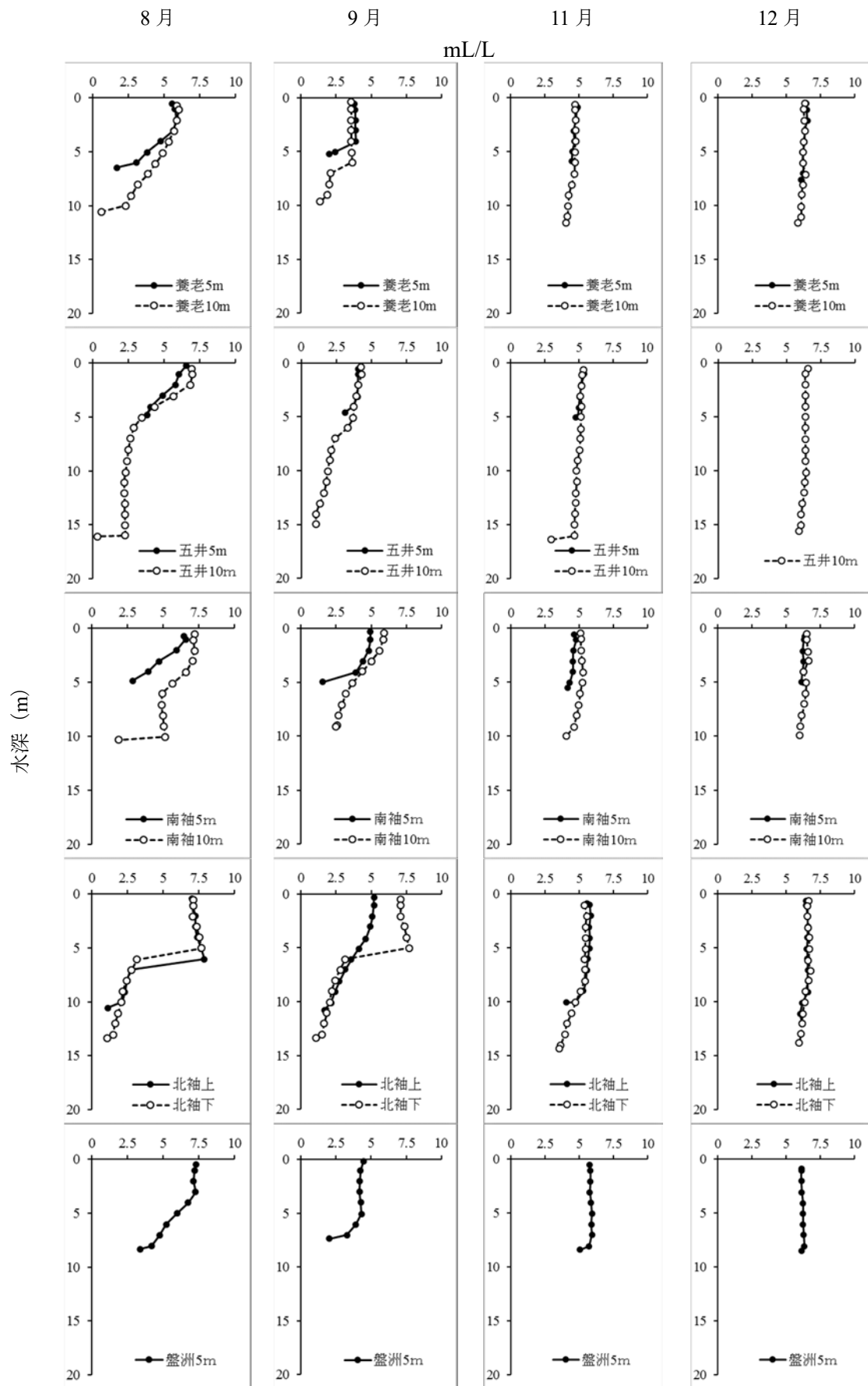
図 2-2-5 つづき. DO の鉛直観測結果(横軸は mL/L) (8、9、11、12 月)
