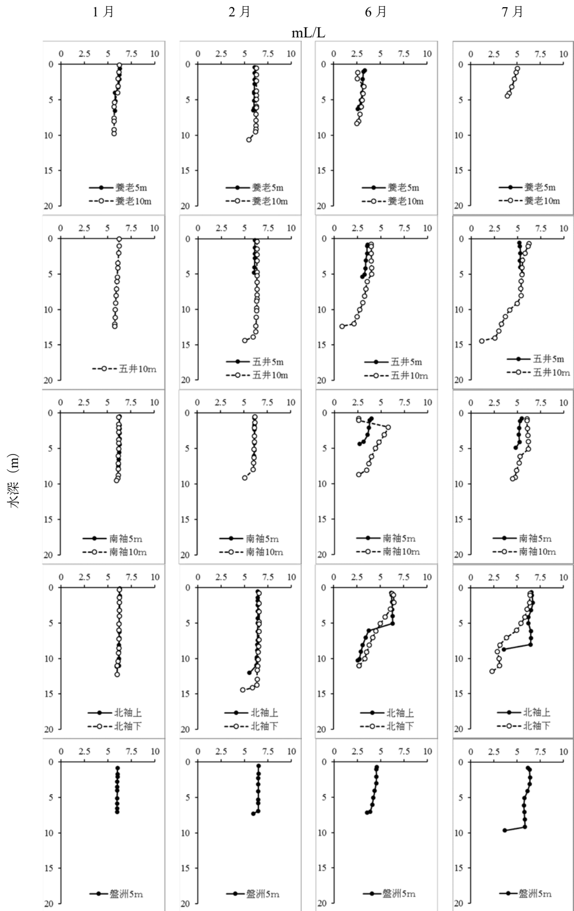
図 2-2-5. DO の鉛直観測結果(横軸は mL/L) (1、2、6、7 月)
