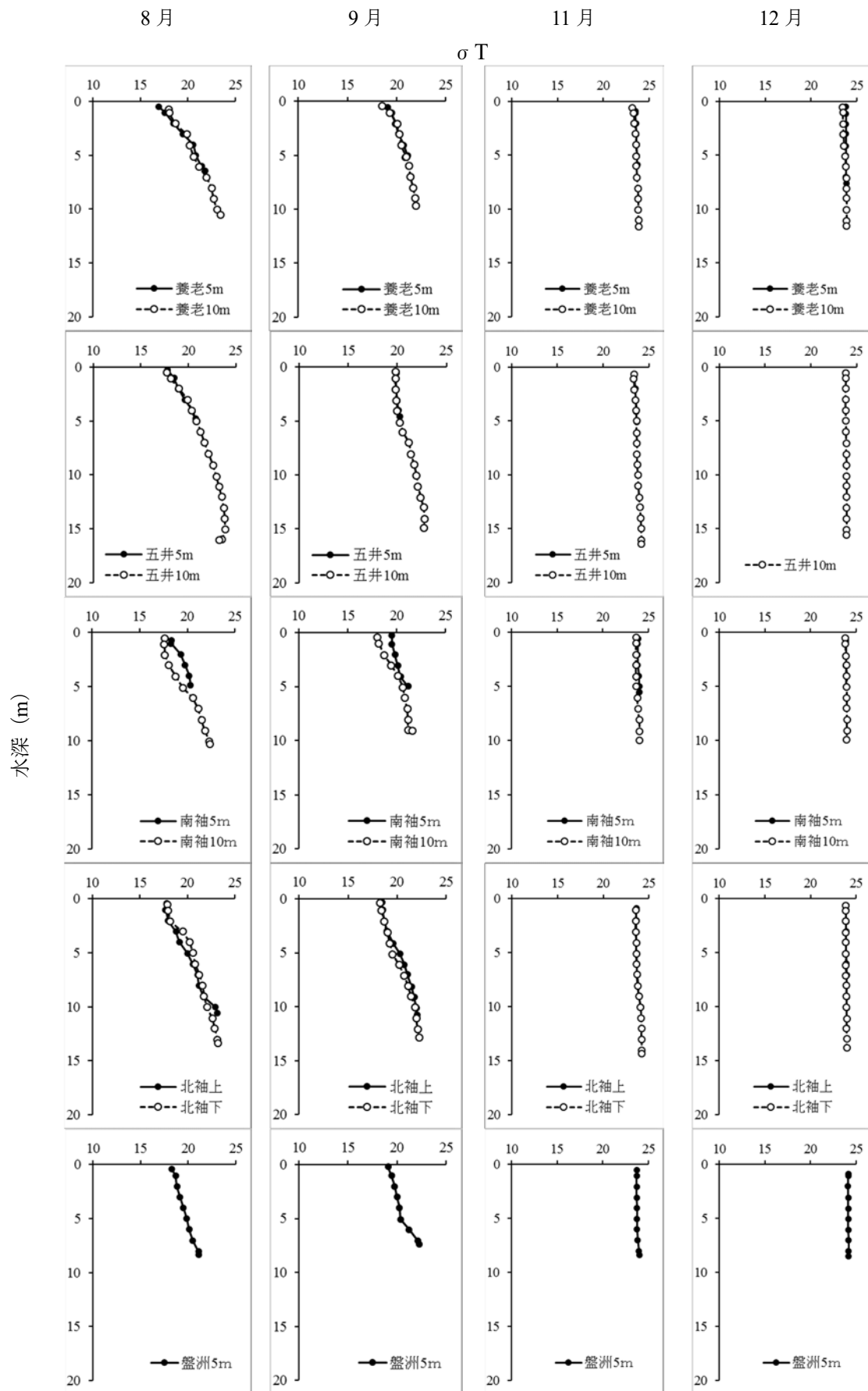
図 2-2-3 つづき. 密度 ( \sigma T ) の鉛直観測結果 (8、9、11、12 月)
