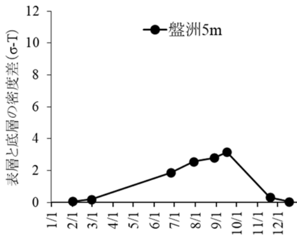
図 2-2-4. 表層と底層の密度 ( \sigma_T ) 差の季節変化
