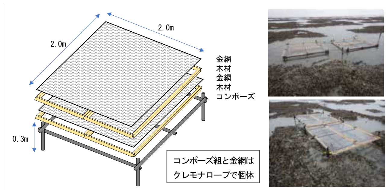
図33 令和3年度の棚式着生材のモデルおよび現地の設置状況
