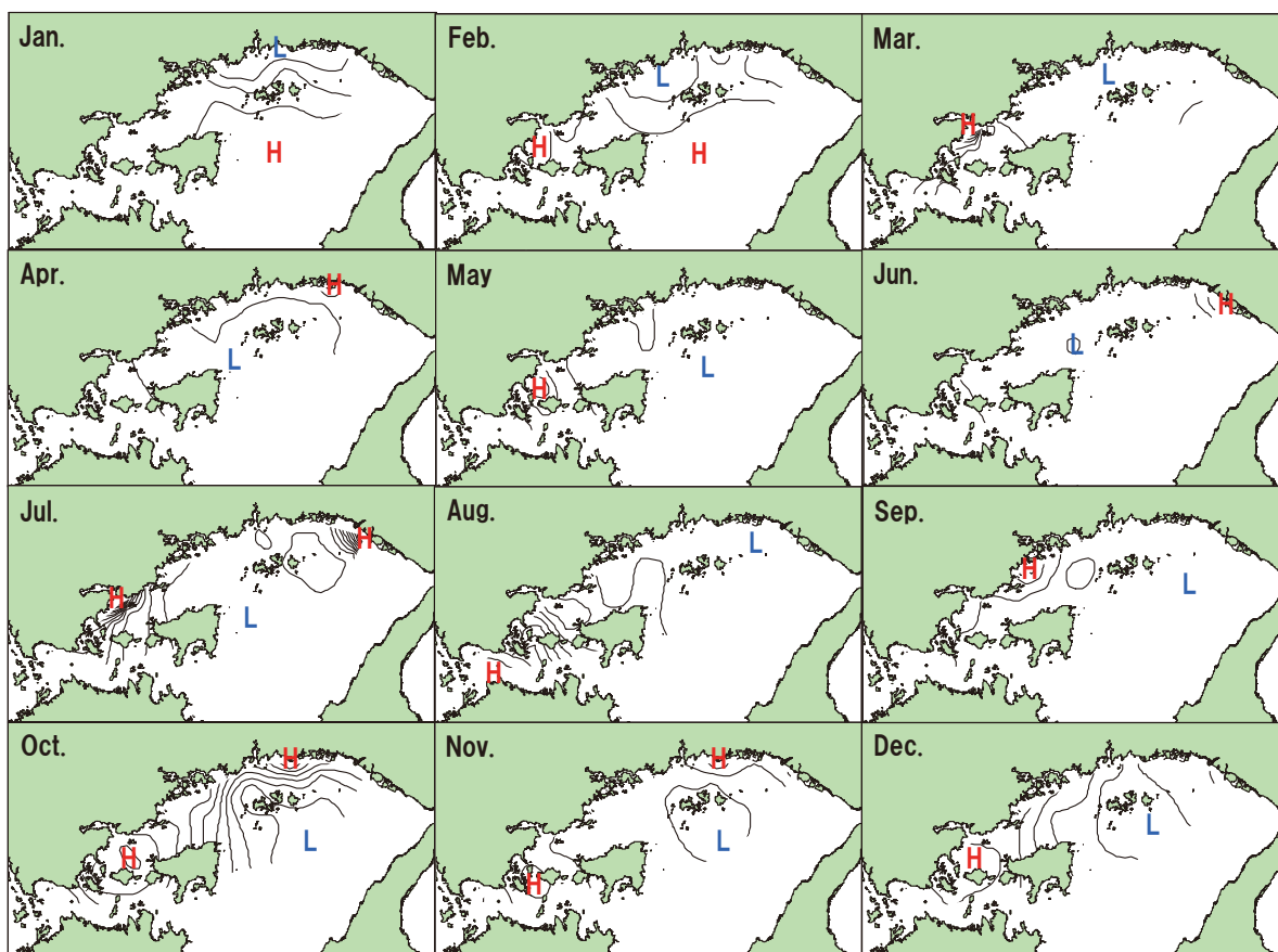
図6 播磨灘北西部の表層 DIN 濃度分布 (2020 年, \mu\text{M} )
