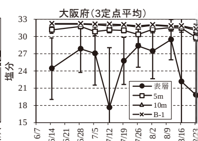
図8 塩分の変動
