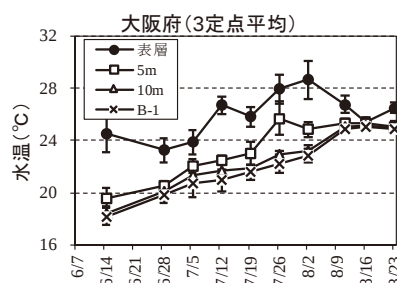
図7 水温の変動(縦バーは標準偏差。以下同じ)
