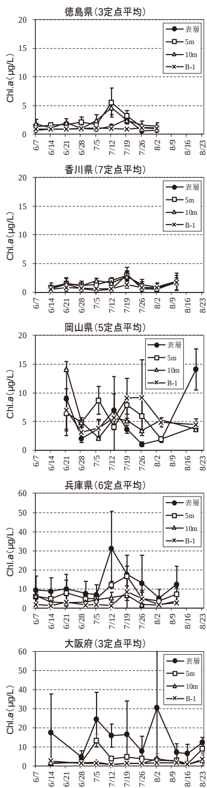
図 13 Chl. a の変動
