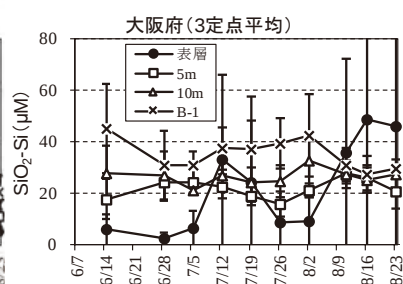
図 12 SiO 2 -Si の変動
