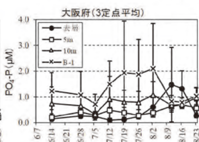
図 11 PO 4 -P の変動
