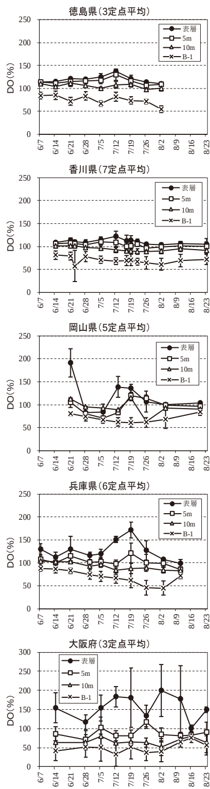
図 14 DO の変動
