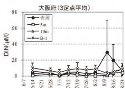
図 10 DIN の変動
