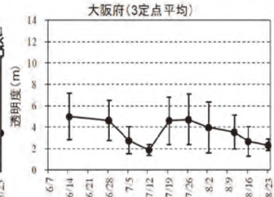
図9 透明度の変動
