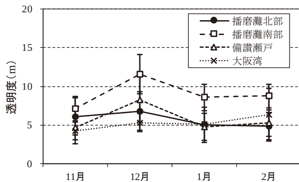
図 28 透明度の変動
