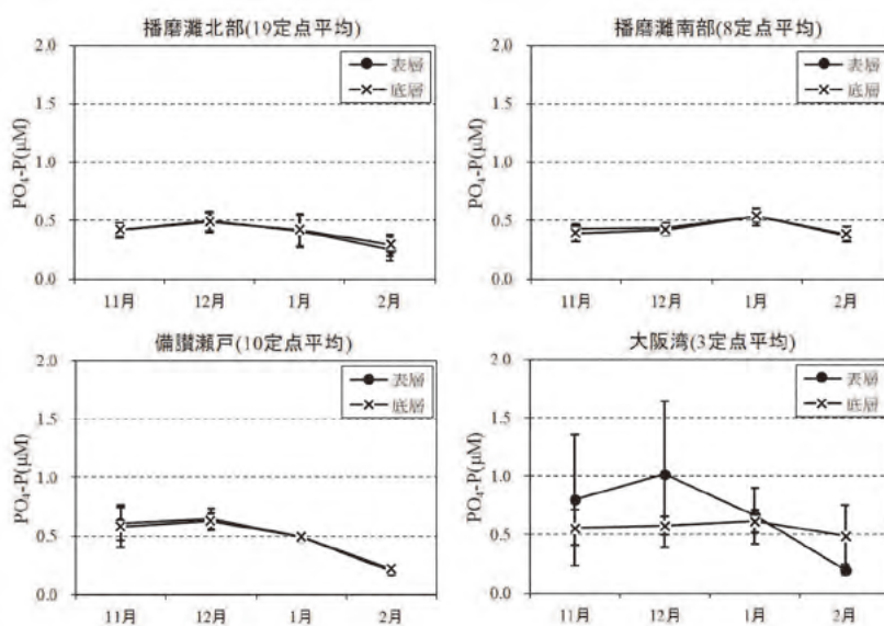
図 30 PO 4 -P の変動
