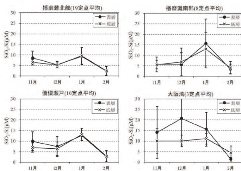
図 31 SiO 2 -Si の変動
