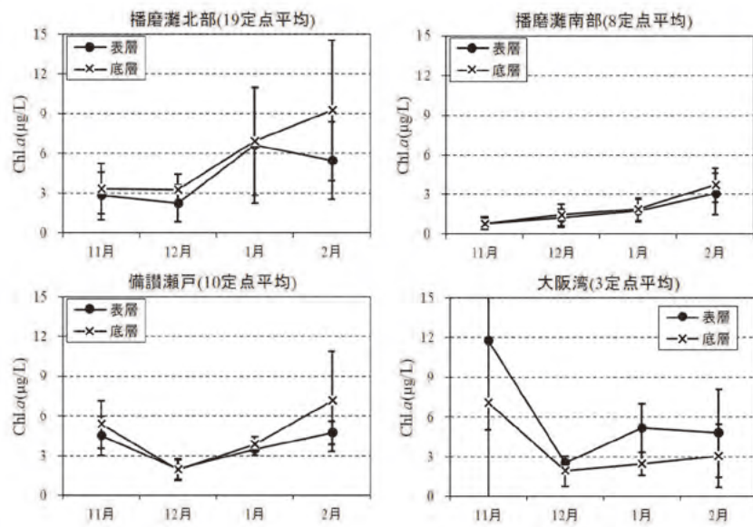
図 32 Chl. a の変動
