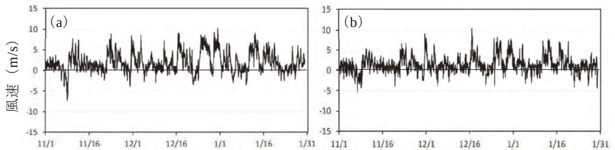
図 34 高松 (a) および姫路 (b) における西風成分の変動 (データは気象庁気象統計情報から引用)
