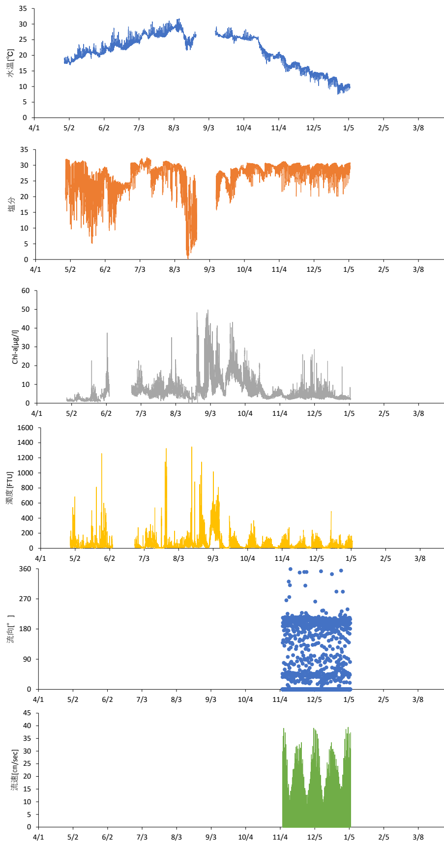
図9 10号地区の連続観測結果(4月～翌年1月)
