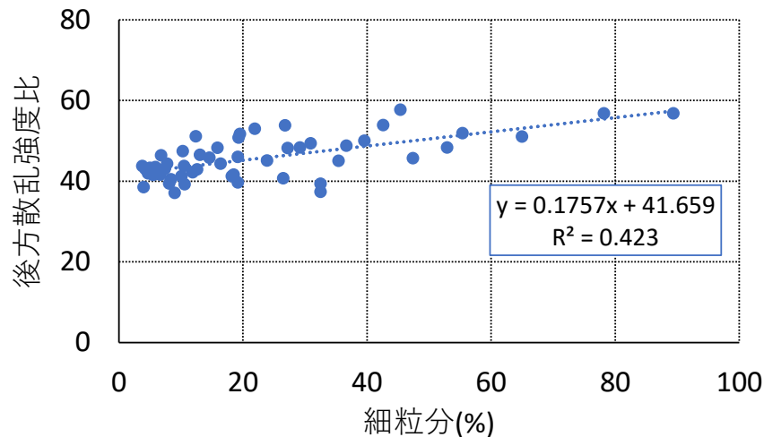
図7 後方散乱強度比と細粒分の相関
