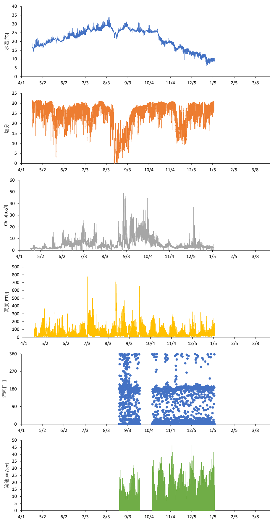
図8 4号地区の連続観測結果(4月～翌年1月)
