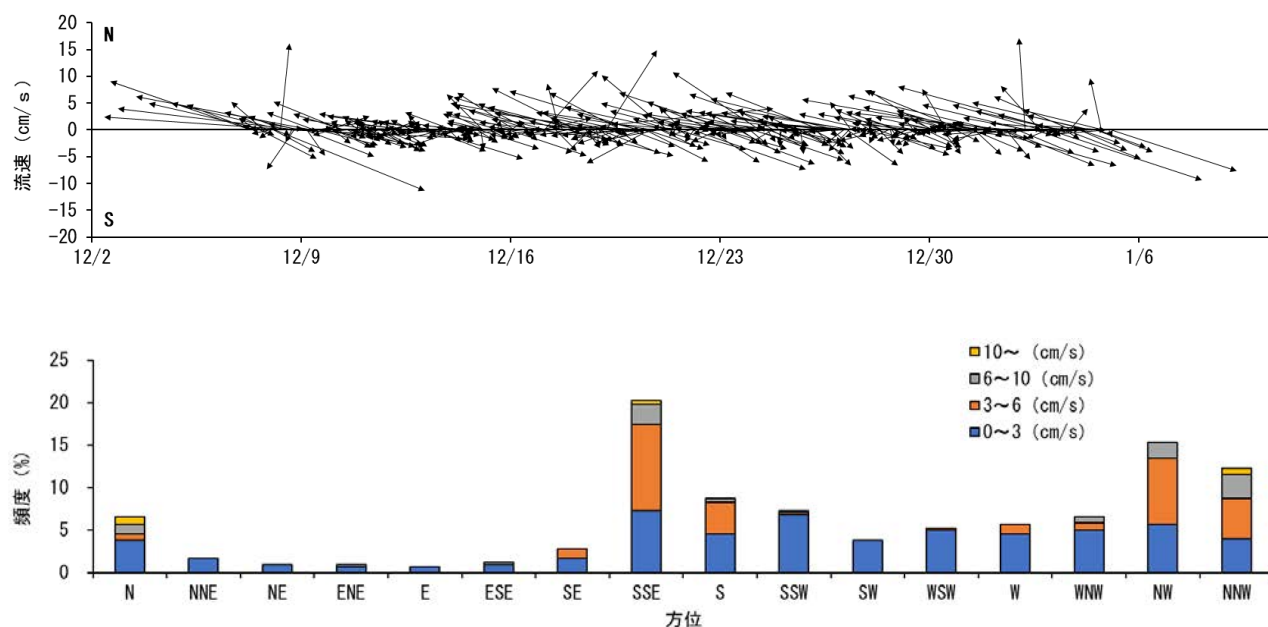
図9 釜漁場流況調査結果_冬季調査（上図：流向・流速、下図：出現頻度）
