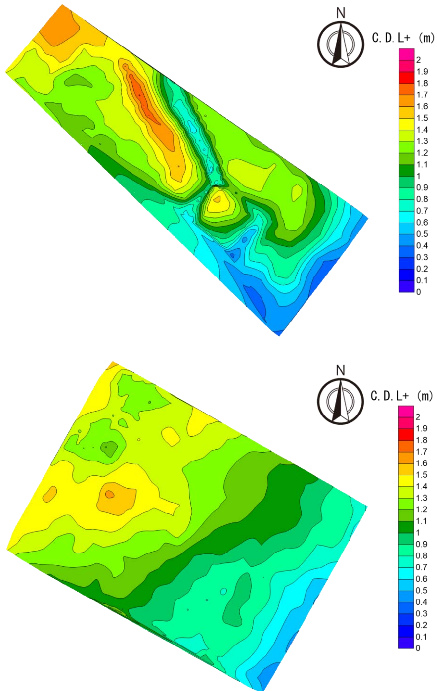
図6 地盤高測量結果（上図：釜漁場、下図：長里漁場）
