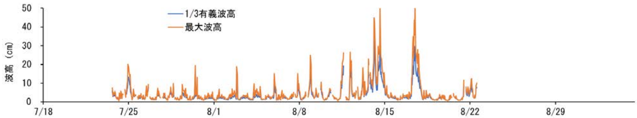
図11 釜漁場波高調査結果_夏季調査
