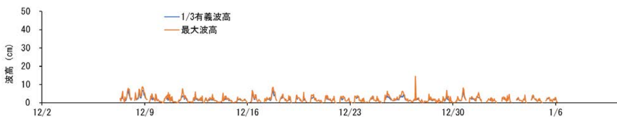
図14 長里漁場波高調査結果_冬季調査結果
