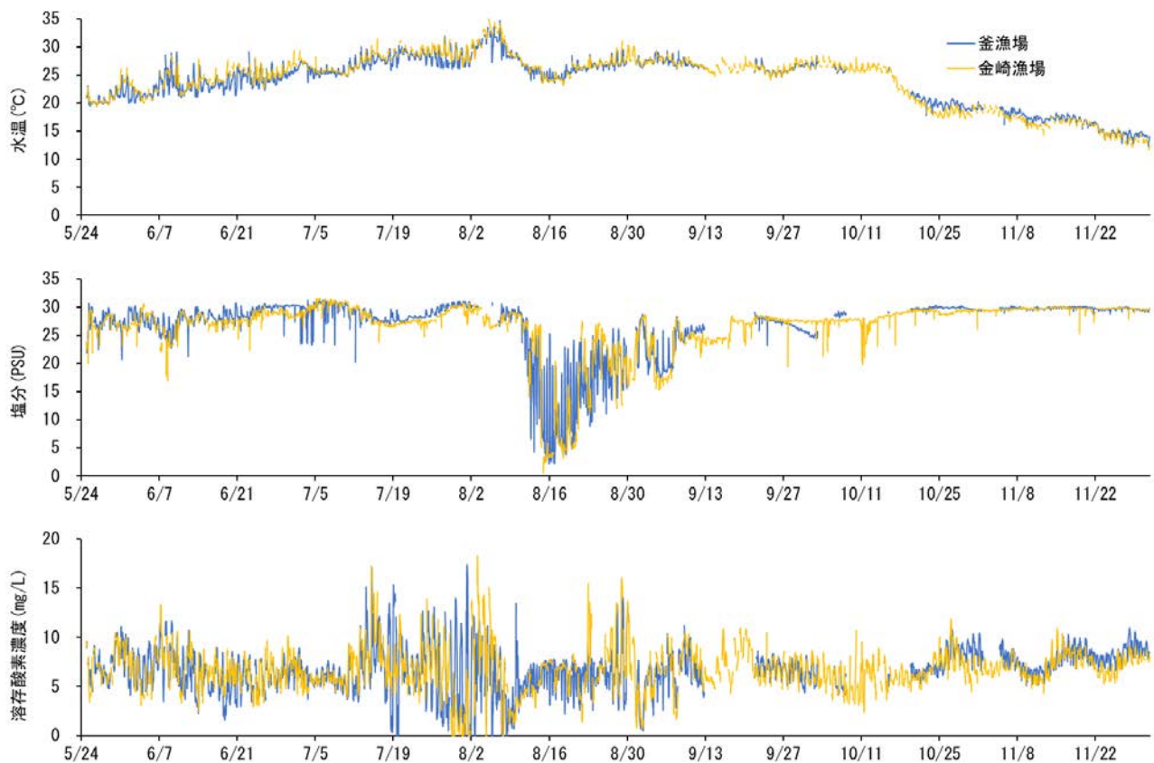
図25 テレメータ観測結果（上図：水温、中図：塩分、下図：溶存酸素濃度）
