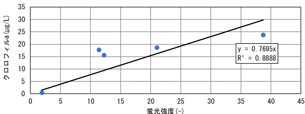
図20 蛍光強度-クロロフィルa 検量線
