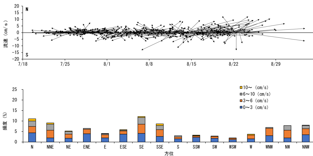
図8 長里漁場流況調査結果_夏季調査（上図：流向・流速、下図：出現頻度）
