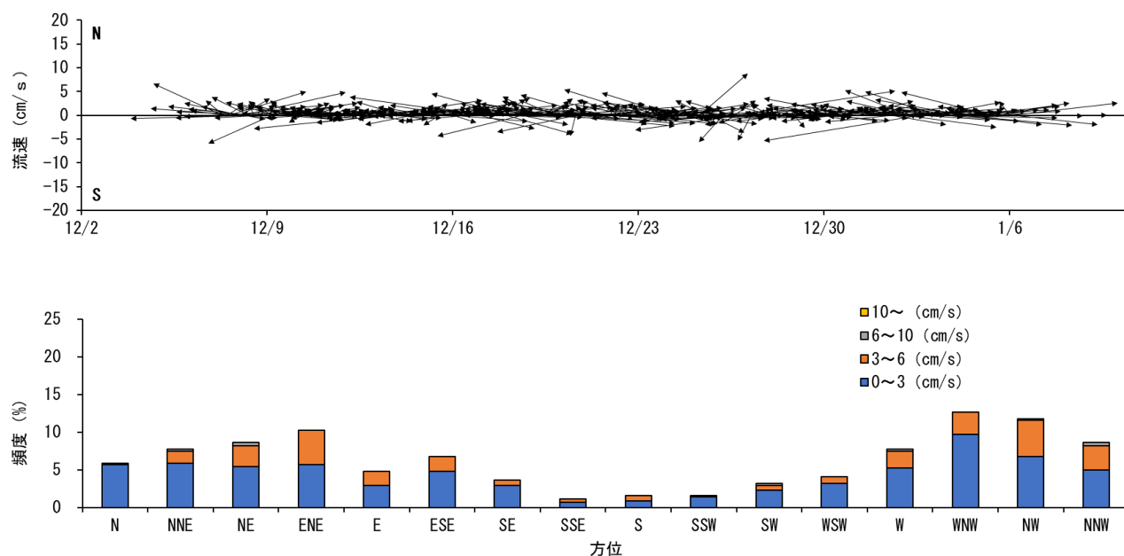
図10 長里漁場流況調査結果_冬季調査（上図：流向・流速、下図：出現頻度）
