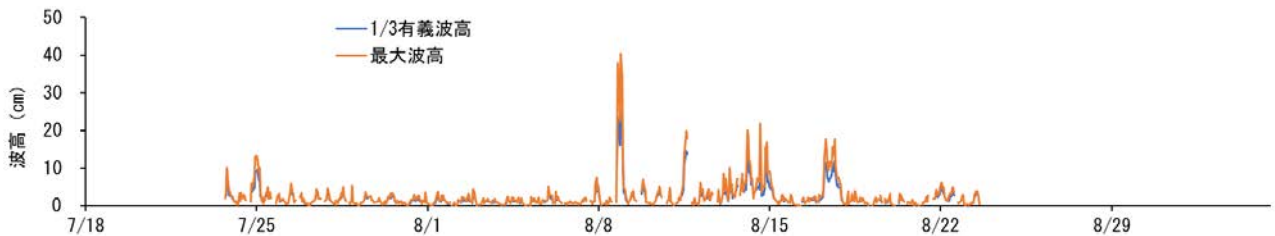
図12 長里漁場波高調査結果_夏季調査
