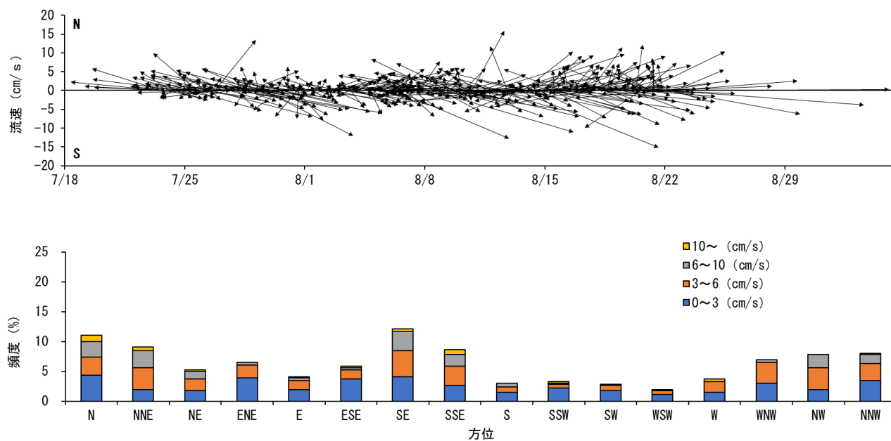
図7 釜漁場流況調査結果_夏季調査（上図：流向・流速、下図：出現頻度）
