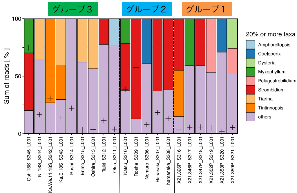
図 11 類型化した 3 グループの特徴：繊毛虫の分類。+ はサンプルにおける繊毛虫の割合。
