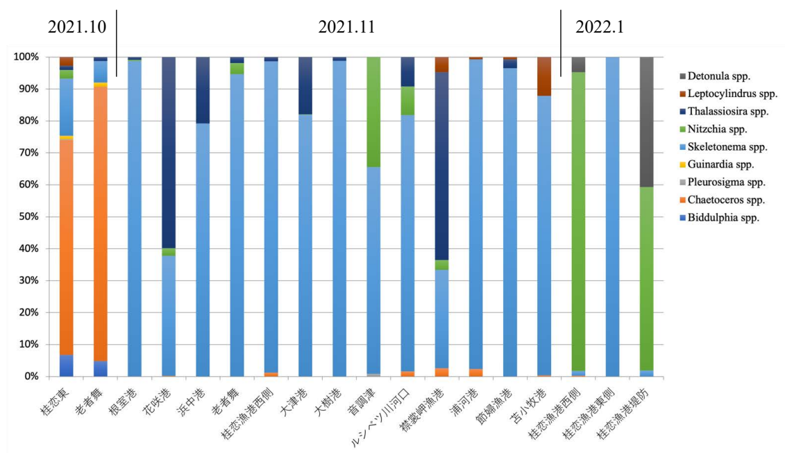
図 13 北海道道東から道南における珪藻類の分布. グラフ上部の日付は、サンプル採取期間.
