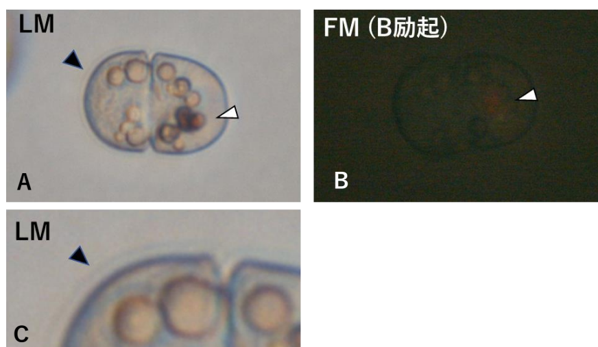
図 14 Karenia selliformis 培養細胞中に観察された一時シスト様の細胞。 A, C: 通常光観察、B: 蛍光観察 (B 励起). 黒矢印: 薄い被膜に覆われている。白 矢印: 細胞内の red body 様粒子。
