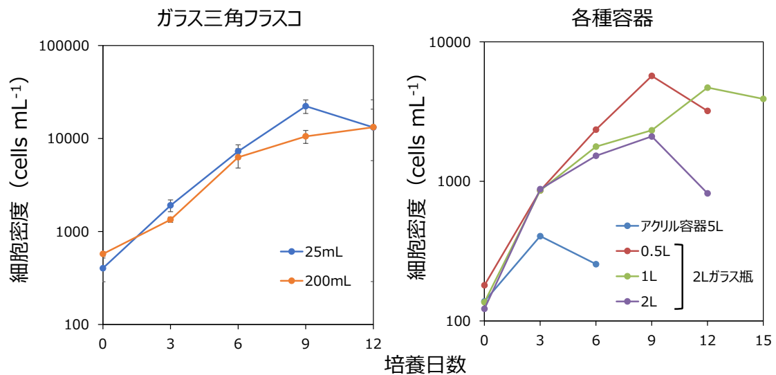
図 12 異なる容量および容器における Karenia selliformis の増殖。
