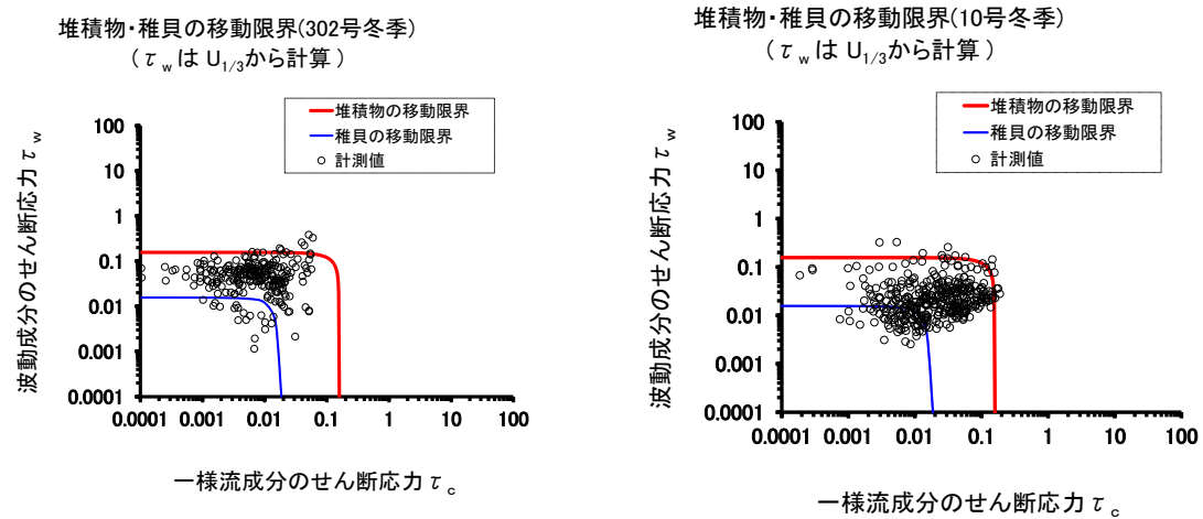
図 15 せん断応力と移動限界判定(冬季)
