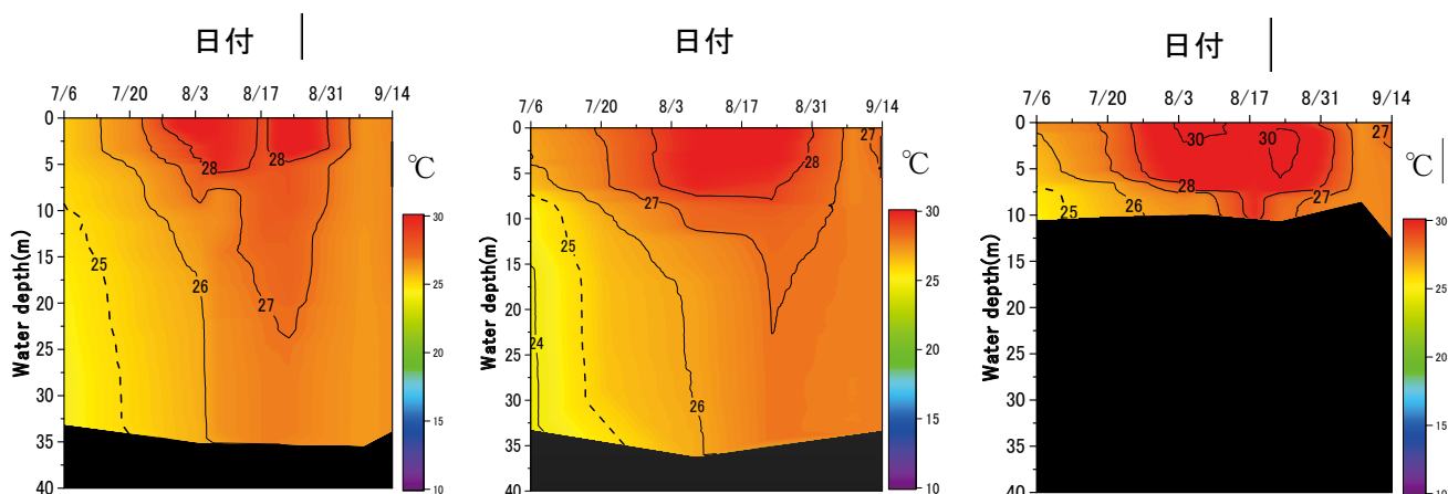
図 1-1-22. 水温の推移(代表 3 点:左図から St.1、St.5、St.9)
