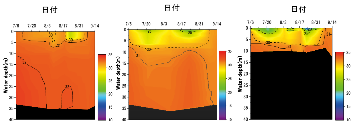
図 1-1-23. 塩分の推移(代表 3 点:左図から St.1、St.5、St.9)
