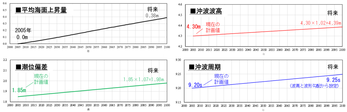
図 3-6.2 外力の経年変化グラフ (B 漁港海岸)
