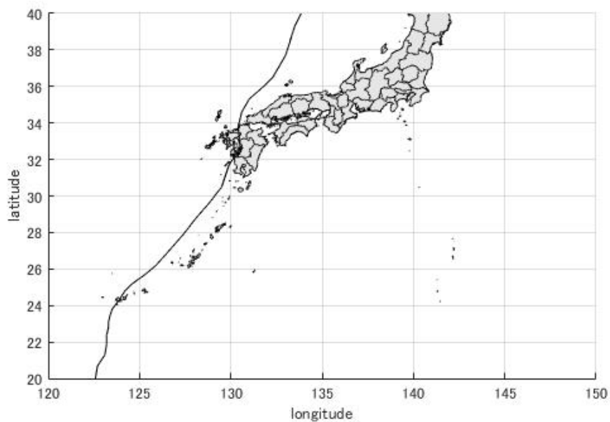
図 3-3.1 2015 年台風第 15 号の経路
