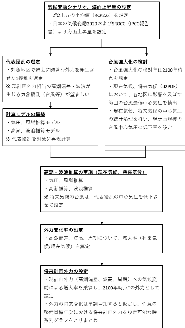
図 3-1.1 外力の将来変化の検討フロー
