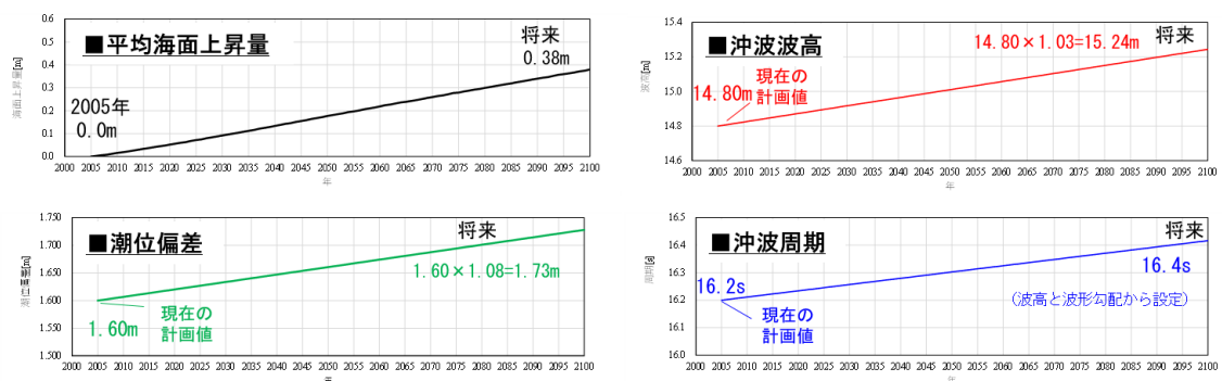
図 3-6.1 外力の経年変化グラフ（A 漁港海岸）
