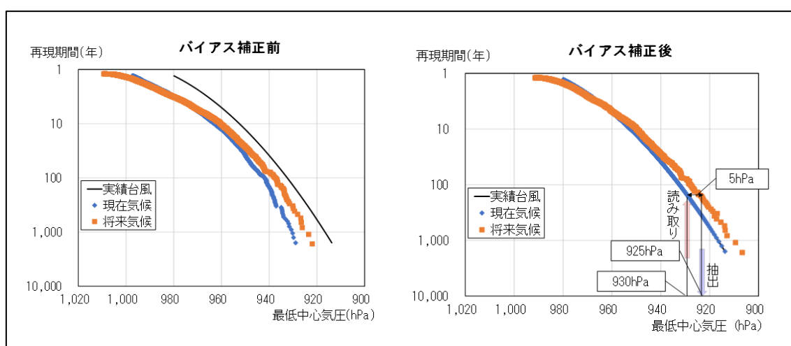
図 3-5.1 最低中心気圧の低下量の設定手順
