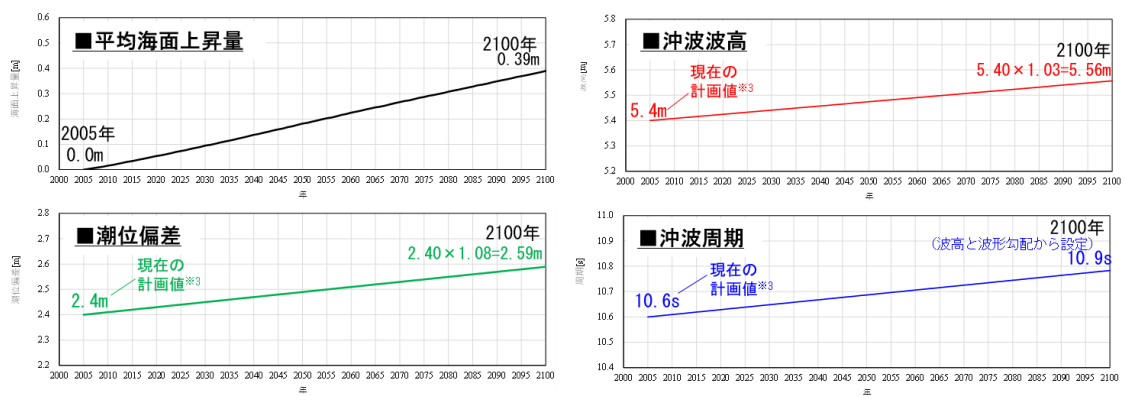
図 3-6.3 外力の経年変化グラフ (C 漁港海岸)
