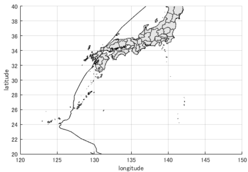
図 3-3.3 1999 年台風 18 号の経路
