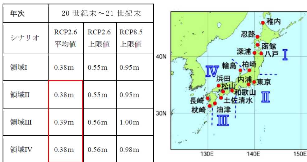
図 3-2.1 21 世紀末における日本沿岸の海面水位の 20 世紀末からの上昇幅
