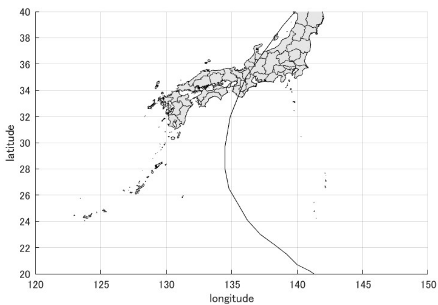
図 3-3.2 伊勢湾台風の経路
