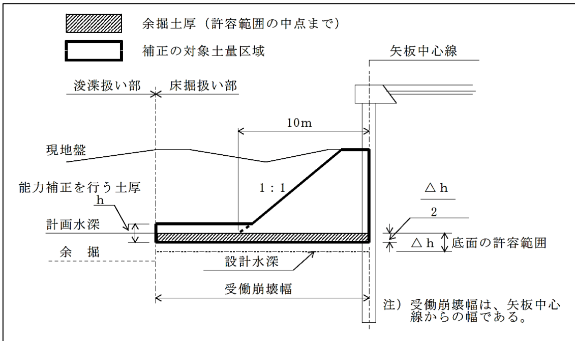
図- 2.7 既設岸壁直近、および受働崩壊幅の範囲内の対象土量区域
