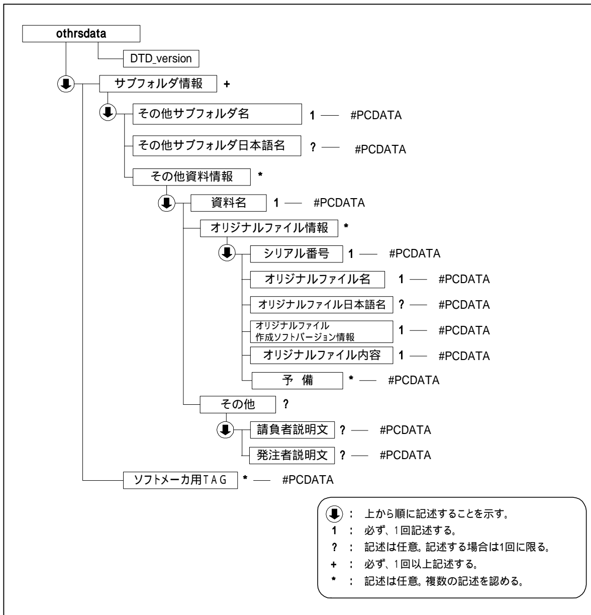
図付 1-4 その他管理ファイルの DTD の構造
