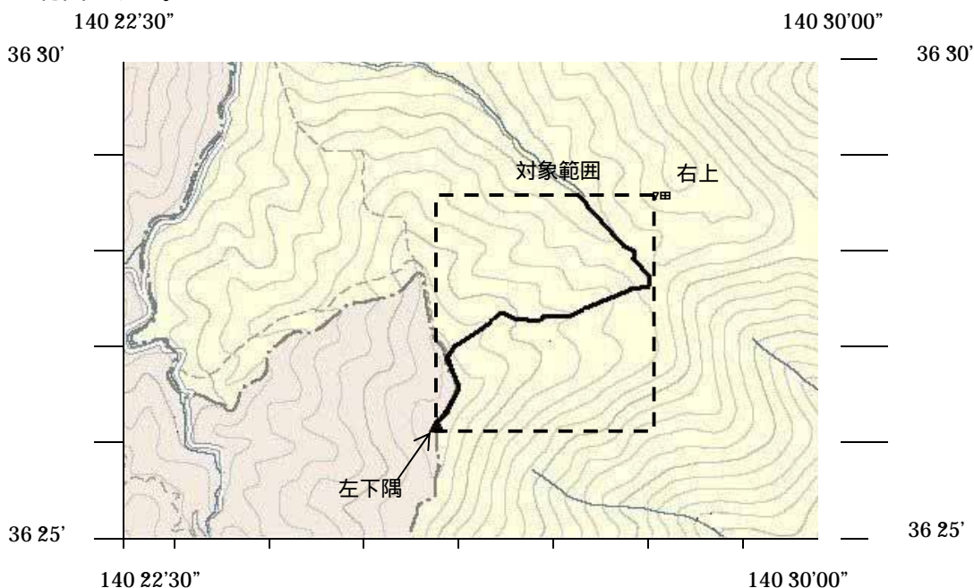
図付 3-6 工事対象範囲の取得方法
