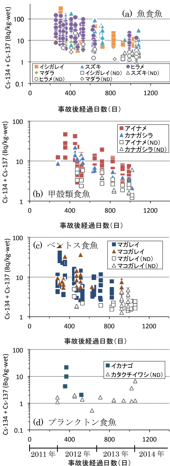
図5. 採餌グループ毎の2011年6月から2014年6月の期間における、Cs濃度の時系列変化 検出限界以下（ND）の個体は白抜きで表す。 また、縦軸のスケールは対数目盛である。
