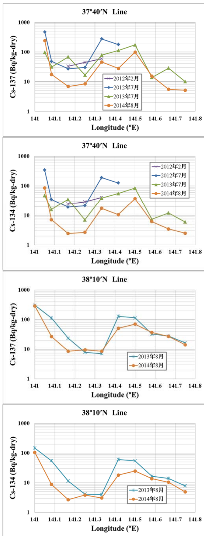
図 3. 福島県北部沖 (37° 40' N:上 2 段) と仙台湾海域 (38° 10' N:下 2 段) それぞれの東西定線における、表層海底土中の Cs-137 と Cs-134 の濃度分布の時系列。期間は 2012 年 2 月から 2014 年 8 月まで。
