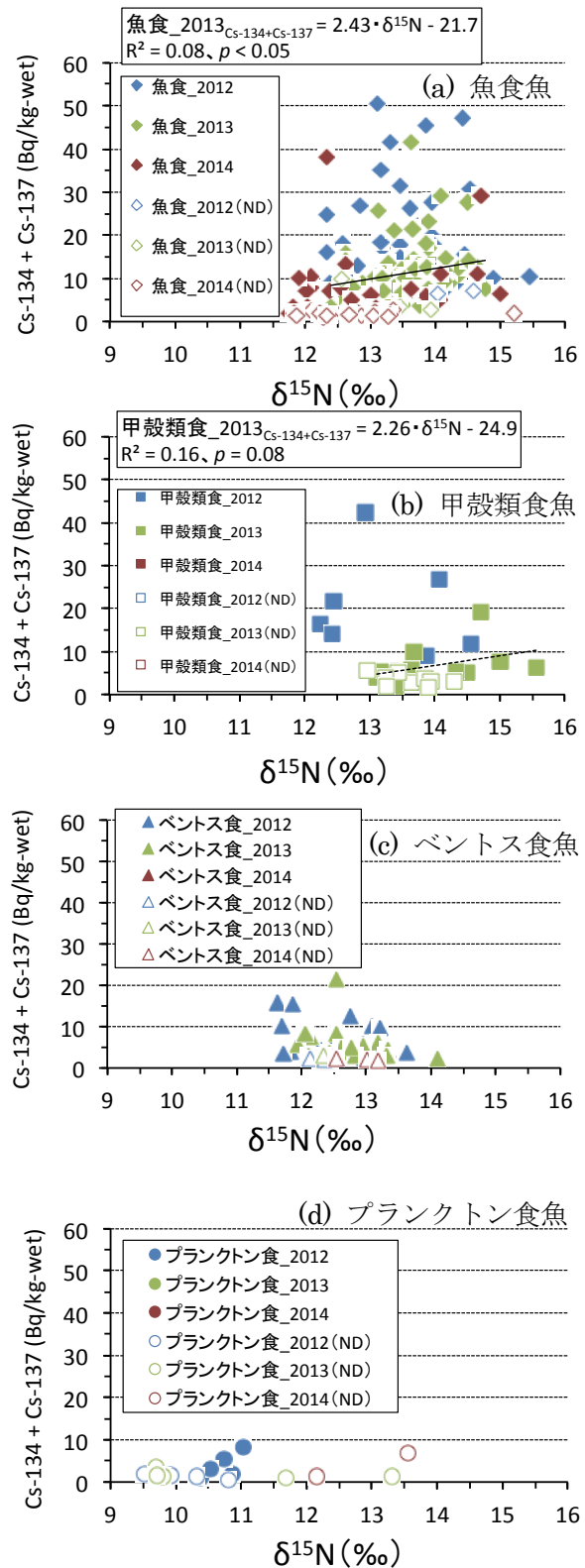
図6. 採餌グループ毎の2012年6月から2014年6月の期間における、 \delta^{15}\text{N} と Cs 濃度との関係 検出限界以下（ND）の個体は白抜きで表す。
