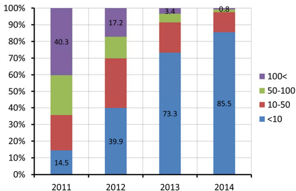
図 4. 2011 年度から 2014 年度までの各年度の福島県沖の底魚類・岩礁性魚類の Cs-134+Cs-137 濃度測定値の 4 階級（ \sim 10\text{Bq/kg-wet} 、 10\sim 50\text{Bq/kg-wet} 、 50\sim 100\text{Bq/kg-wet} 、 100\text{Bq/kg-wet}\sim ）の出現頻度分布。
