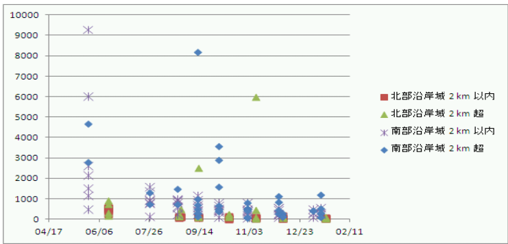
図 1. 福島県沿岸域における平成 23 年 4 月以降の海底土の放射性セシウムの濃度 (Bq/kg-dry) (東電福島第一原発の南北と沖合 2km を境にデータを区分)
