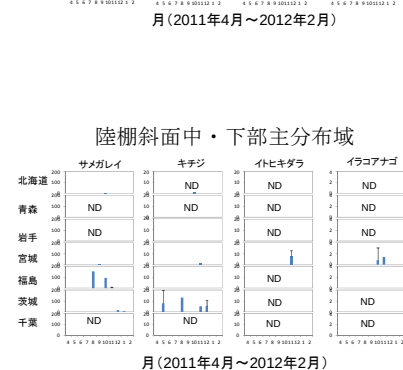
図 5. 県別、月別の主要水産生物の放射性セシウム濃度
