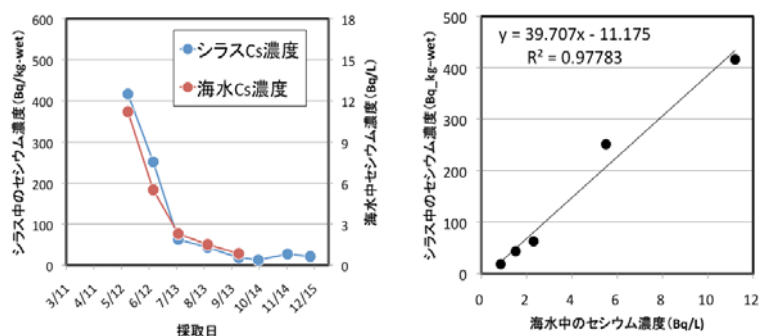
図2 福島県海域で採取されたシラスおよび海水の放射性セシウム濃度の経時変化（a）ならびに8月以降の海水とシラスにおける放射性セシウム濃度の関係（b）
