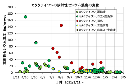
図3 カタクチワシの放射性セシウム濃度の経時変化
