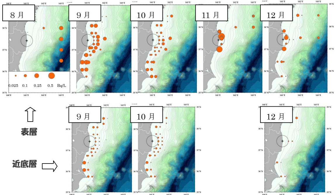
図 2. 東北沖合域における表層（上段）と海底付近（下段）の海水中的 Cs-137 の月毎の濃度分布。
