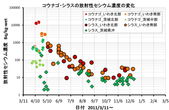
図1 福島県沖および茨城県沖のコウナゴ・シラスの放射性セシウム濃度の経時変化
