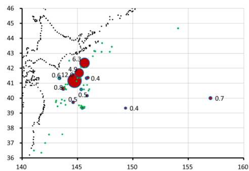
図4 サンマの放射性セシウム濃度測定結果 (Bq/kg-wet)。緑点は検出限界未満
