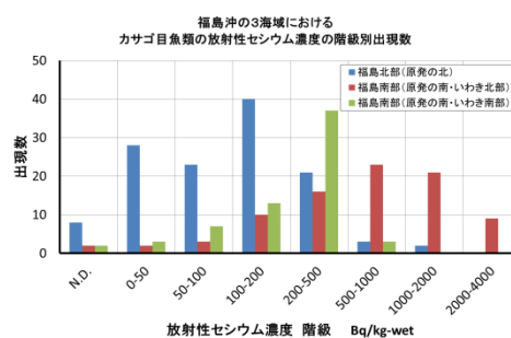
図 2 カサゴ目魚類（メバル、アイナメ等）の福島沖 3 海域での放射性セシウム濃度の出現頻度分布
