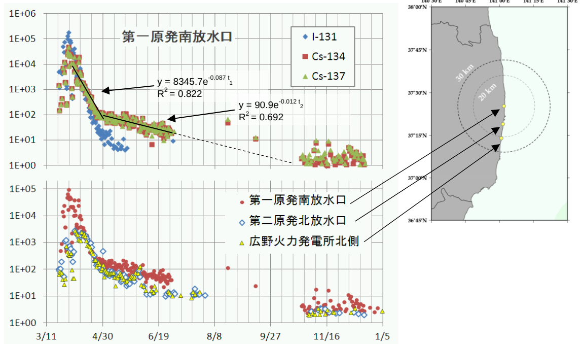
図 1. (上段) 第一原発の南放水口における海水中的各放射性核種濃度の時系列。Cs-137 について、 3/31 < t_1 < 4/30 と 5/1 < t_2 < 7/1 の区間で、時間（日数）に依存する濃度値の近似指数関数を黒線で示す。 (下段) 第一原発、第二原発、火力発電所付近の放射性セシウムの濃度時系列。
