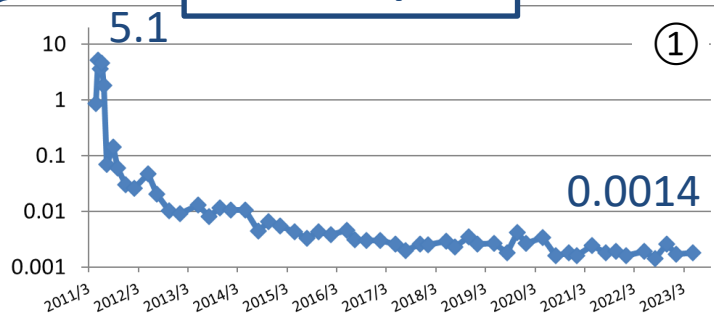
海水(Bq/L)
