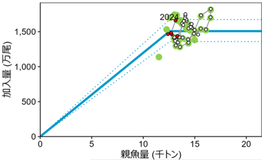
図6 再生産関係
