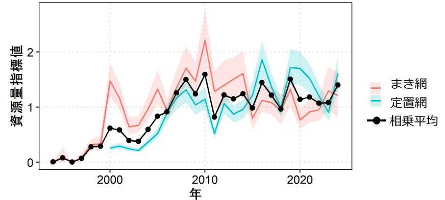
図3 資源量指標値の推移
