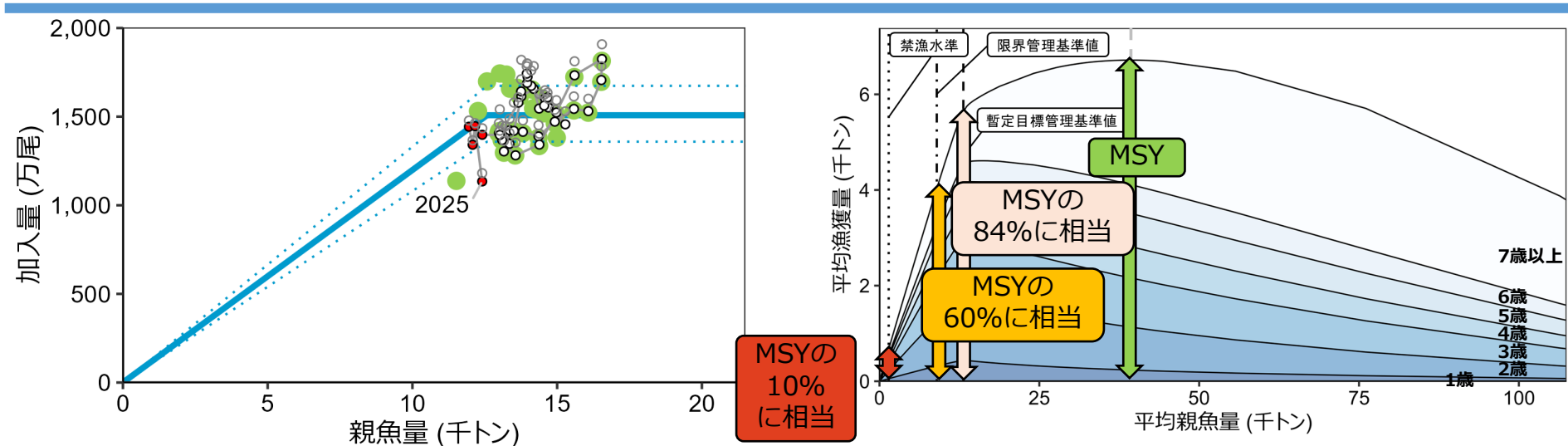
図6 再生産関係
