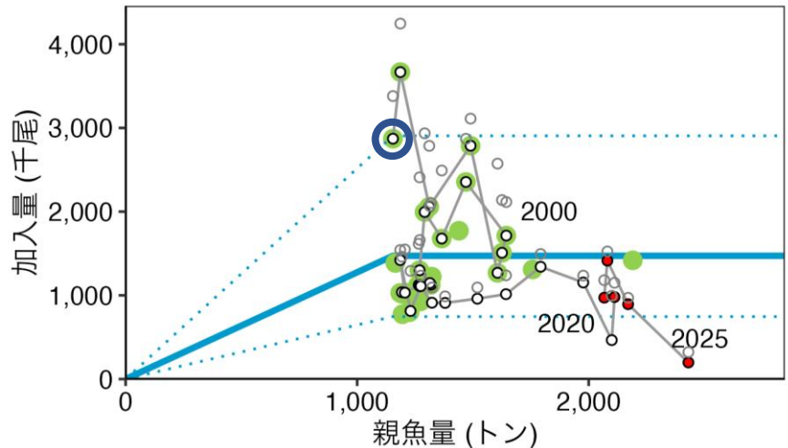
図6 再生産関係
