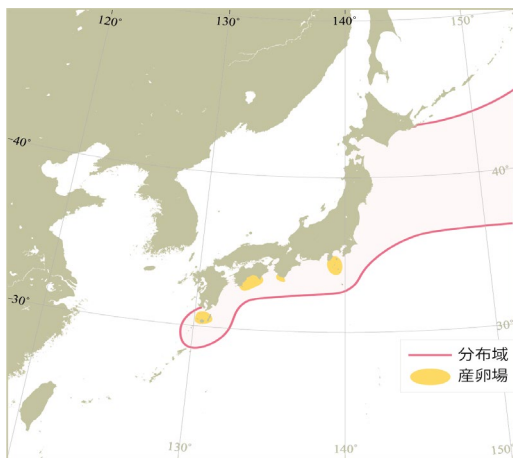
図1 分布図
