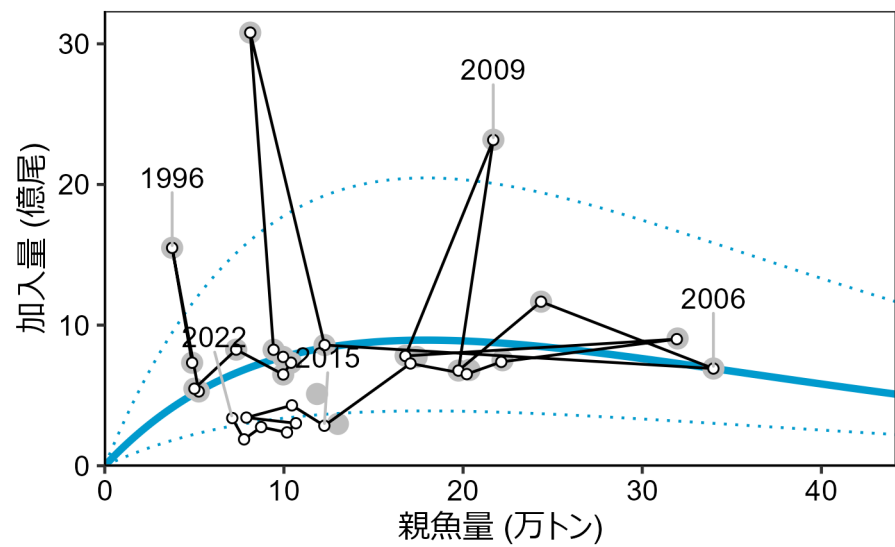
図6 再生産関係
