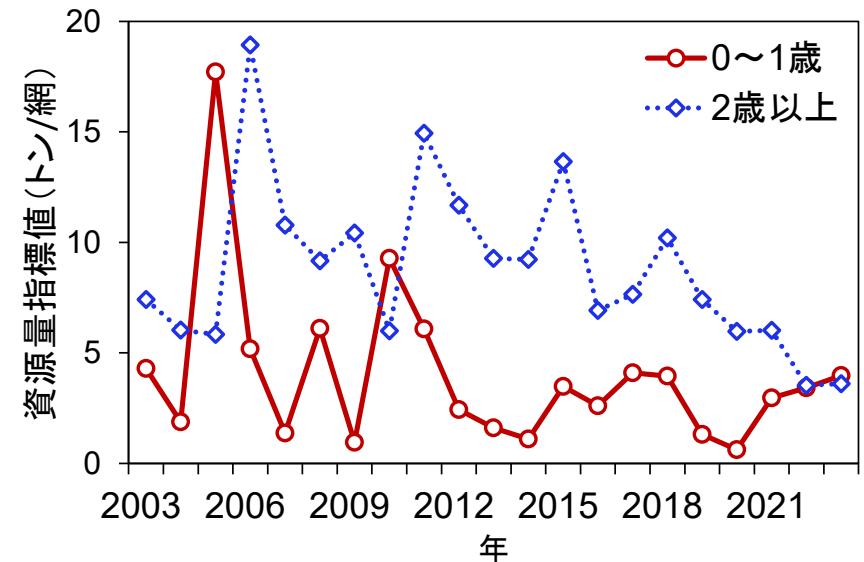
図5 年齢別資源量指標値の推移（枕崎中まき）
