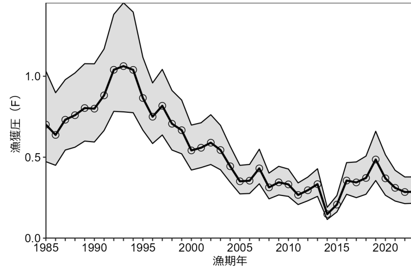
図4 漁獲圧の推移（灰色の網掛けは90%信頼区間）
