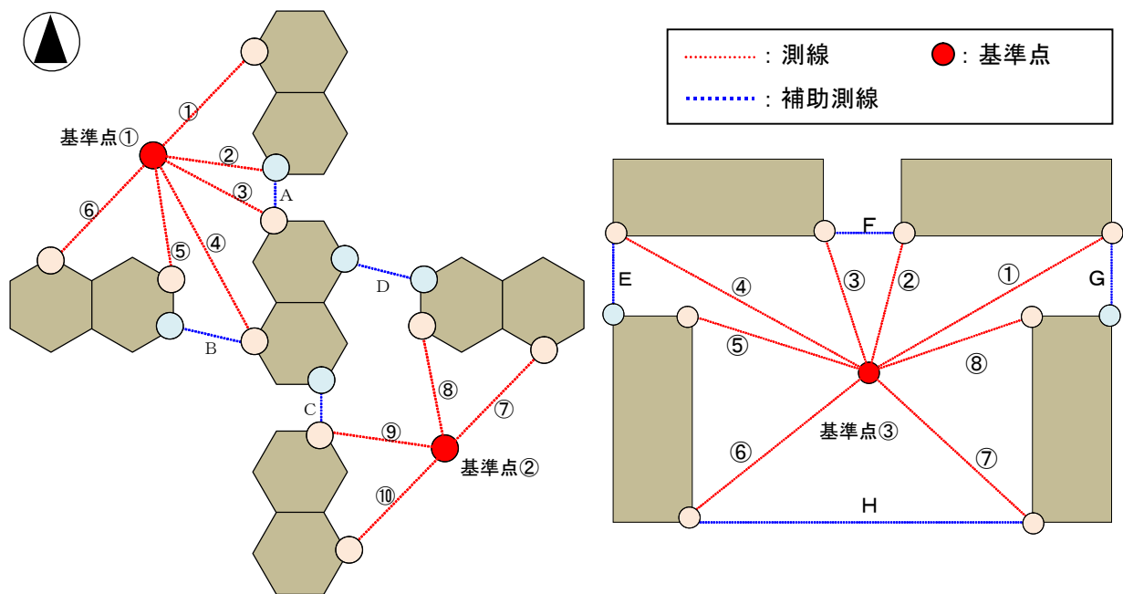
図-IV.1.2.16 安定性確認の計測位置図
