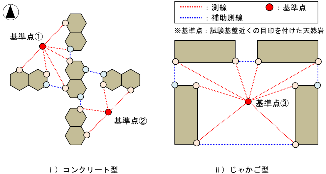
図-IV.1.1.5 計測位置図
