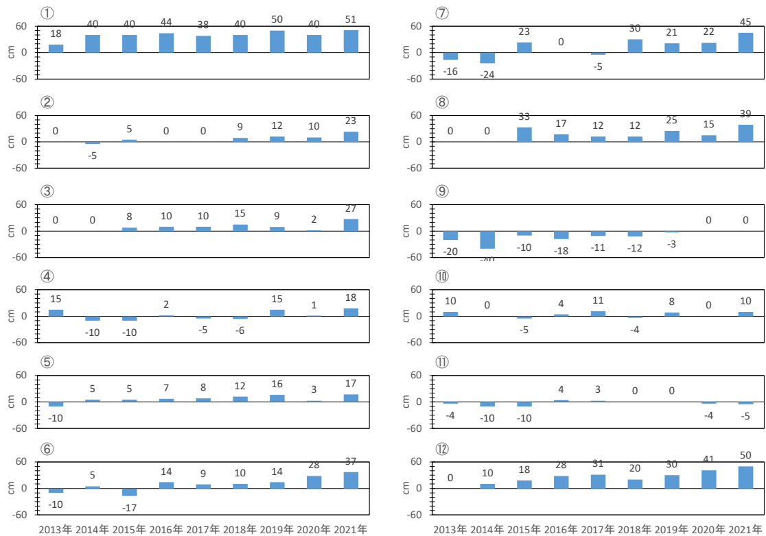
図-IV.1.2.15 中間育成施設周辺の堆積砂厚の推移（じゃかご型）
