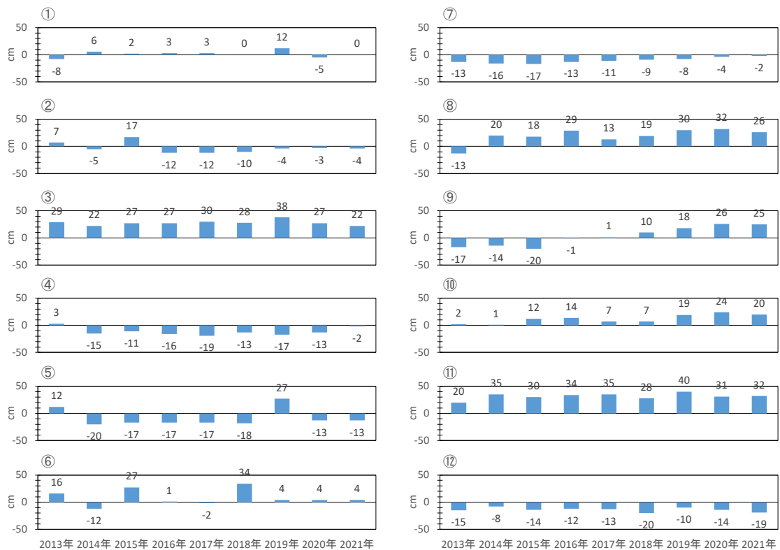
図-IV.1.2.14 中間育成施設周辺の堆積砂厚の推移（コンクリート型）
