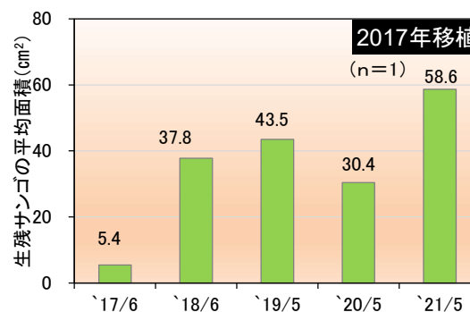
図-IV.1.2.2 2017年移植サンゴの成長面積
