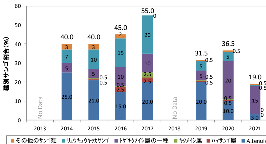
図-IV.1.2.5 対照区ノル(A6)コドラート調査におけるサンゴ被度経年変化
