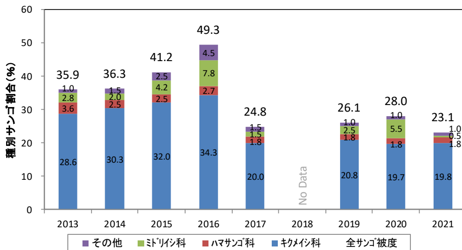
図-IV.1.2.4 対照区ノル(A6)全体でのサンゴ被度経年変化
