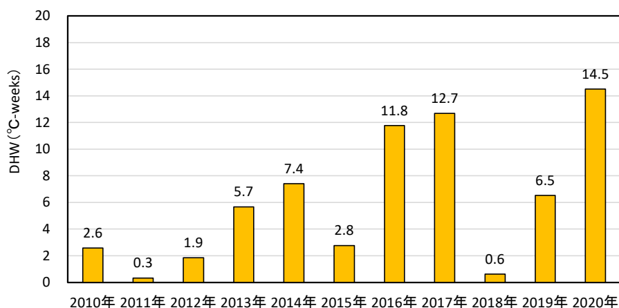
図-IV.1.3.7 DHWの推移（2010～2020年）
