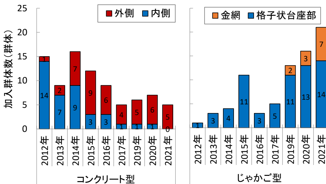
図-IV.1.2.19 新規加入群体数の推移
