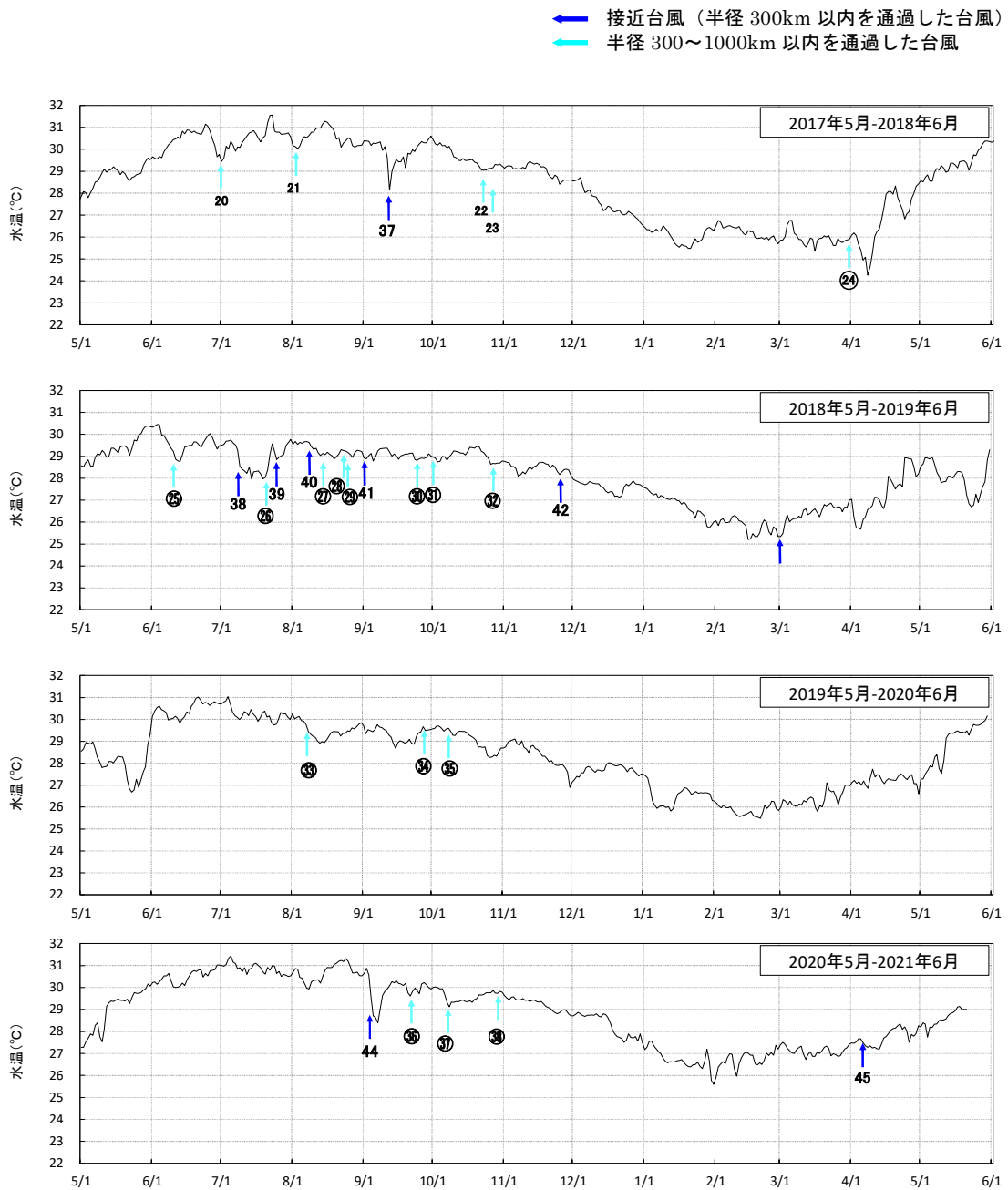
図-IV. 1. 3. 3(3) 過年度における礁内日平均水温の変化（2017年5月～2021年6月） ※台風のNo.および情報は表-IV. 1. 1. 3. 3、表-IV. 1. 1. 3. 4に示す通り
