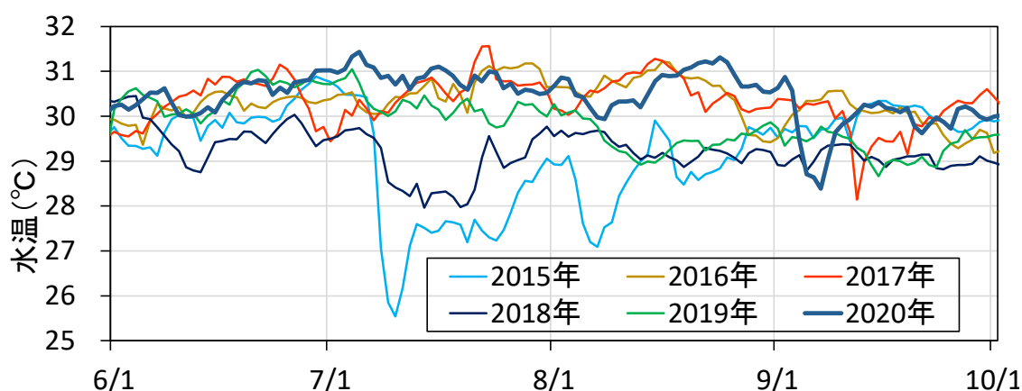
図-IV.1.3.1 6～9月の中間育成施設内の日平均水温変動（6ヶ年分の比較）
