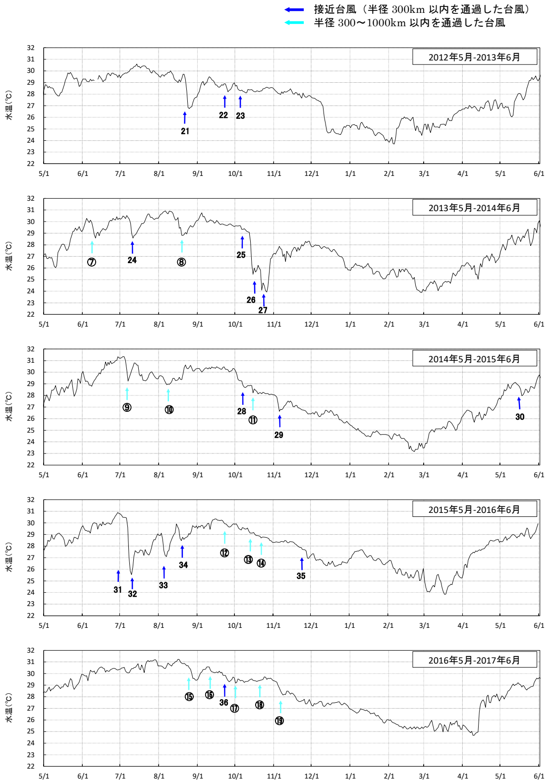
図-IV.1.3.3(2) 過年度における礁内日平均水温の変化（2012年5月～2017年6月） ※台風のNo.および情報は表-IV.1.1.3.3、表-IV.1.1.3.4に示す通り
