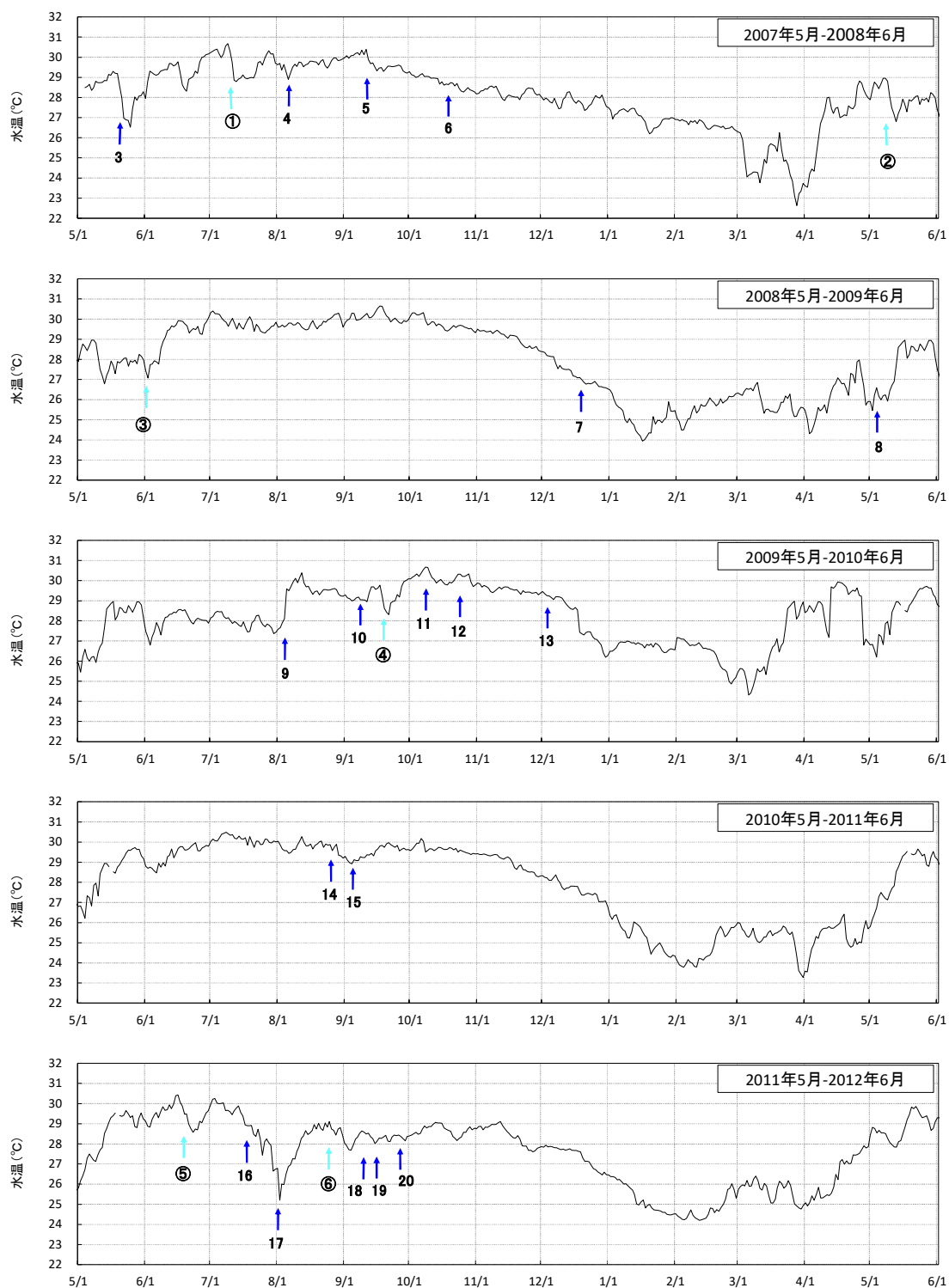
図-IV.1.3.3(1) 過年度における礁内日平均水温の変化 (2007年5月～2012年6月) ※台風のNo.および情報は表-IV.1.1.3.3、表-IV.1.1.3.4に示す通り
