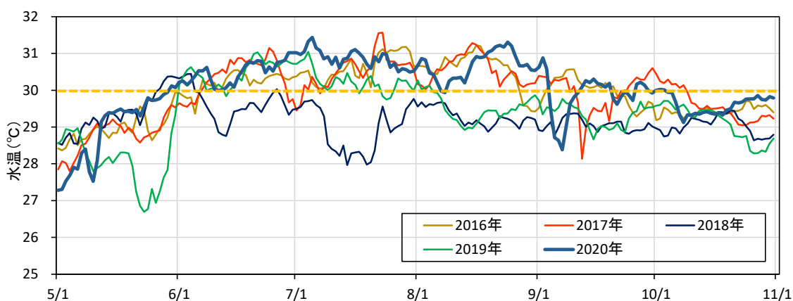
図-IV.1.3.5 5～11月の礁内日平均水温変動（5ヵ年分の比較）
