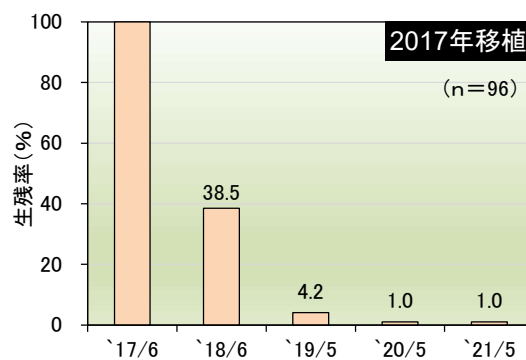
図-IV.1.2.1 2017年6月移植の生残率
