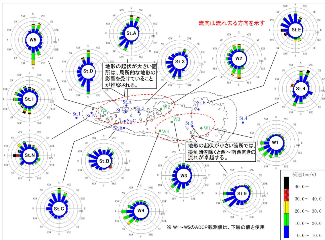
図-Ⅲ. 2. 1. 7 サンゴ産卵時期（5～7月）の礁内の流向・流速頻度
