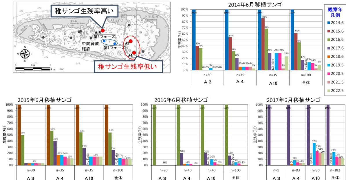
図-Ⅲ. 2. 1. 5 移植サンゴの生残率の推移
