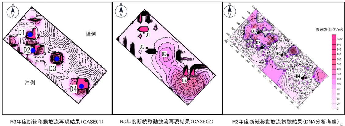
図-Ⅲ. 2. 1. 5 R3 年度再現計算結果
