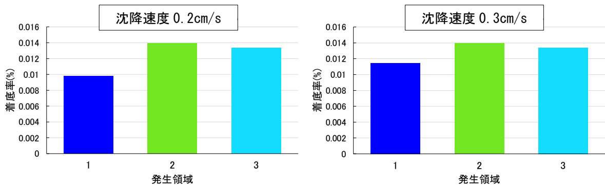
図-Ⅲ. 2. 2. 9 検討 1 の領域毎の着底率 (21 年平均 ※2013 年を除外)
