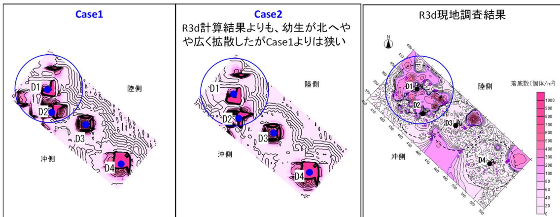
図-Ⅲ. 2. 1. 3 R3 年度の再現計算検証結果②（断続移動式放流）
