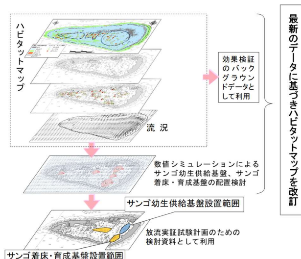
図-III. 2.1.1 ハビタットマップ改訂のイメージ
