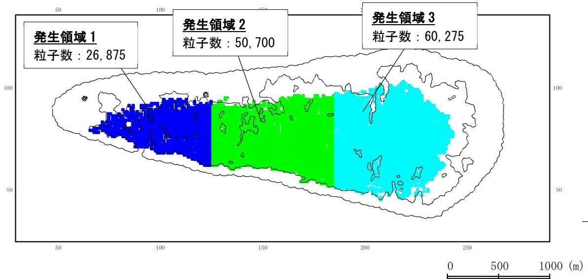
図-Ⅲ. 2. 2. 8 検討 1 における粒子の初期投入箇所および粒子数
