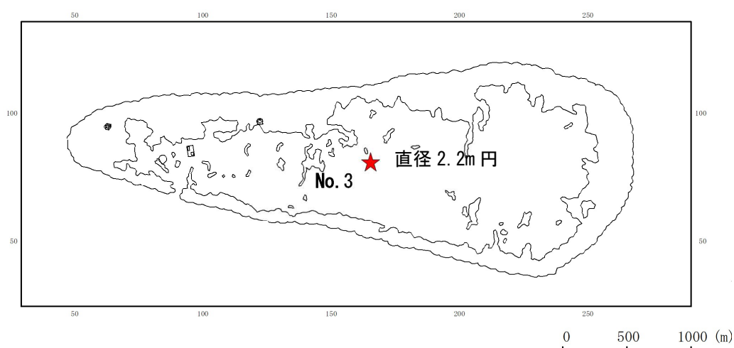
図-Ⅲ.2.2.13 粒子の初期投入箇所
