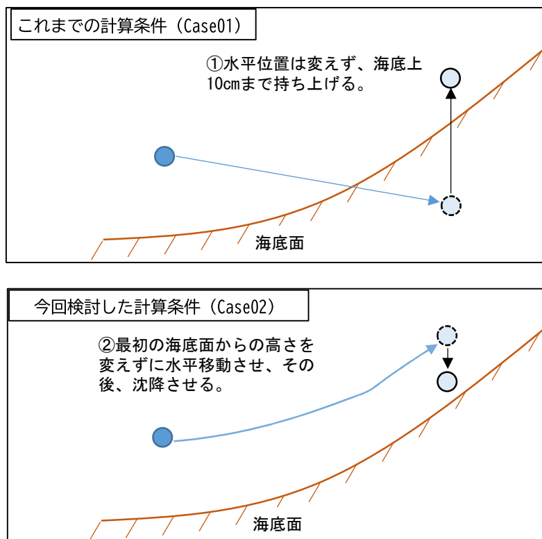
図-Ⅲ. 2. 1. 4 幼生の鉛直方向への移動計算方法概要
