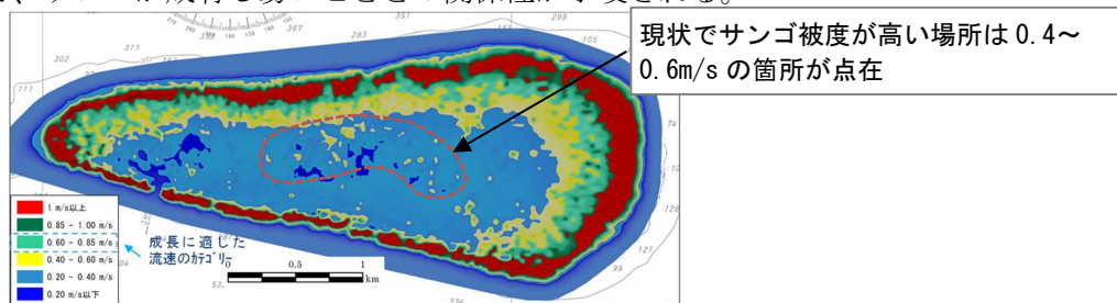
図-Ⅲ. 2. 1. 10 底面軌道流速振幅の分布図
