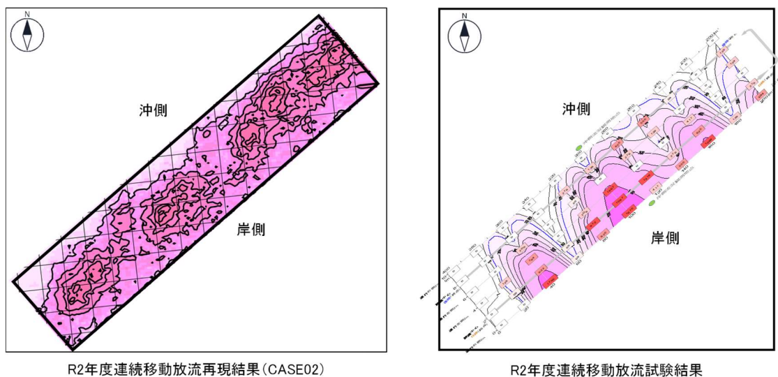
図-Ⅲ. 2. 1. 6 R2 年度再現計算結果
