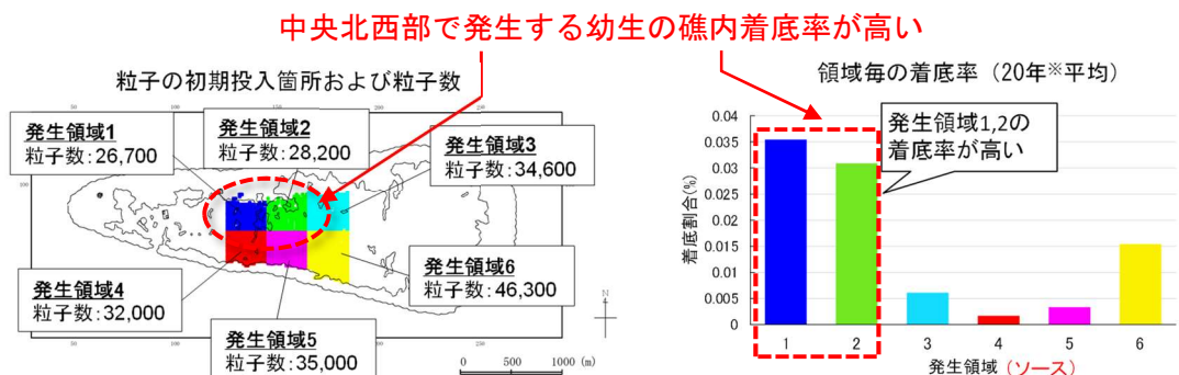
図-Ⅲ. 2. 1. 12 検討領域・粒子数及び領域毎の着底数、着底割合
