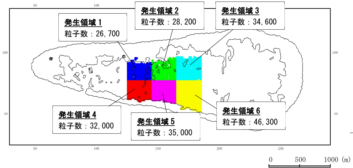
図-III.2.2.10 検討 2 における粒子の初期投入箇所および粒子数
