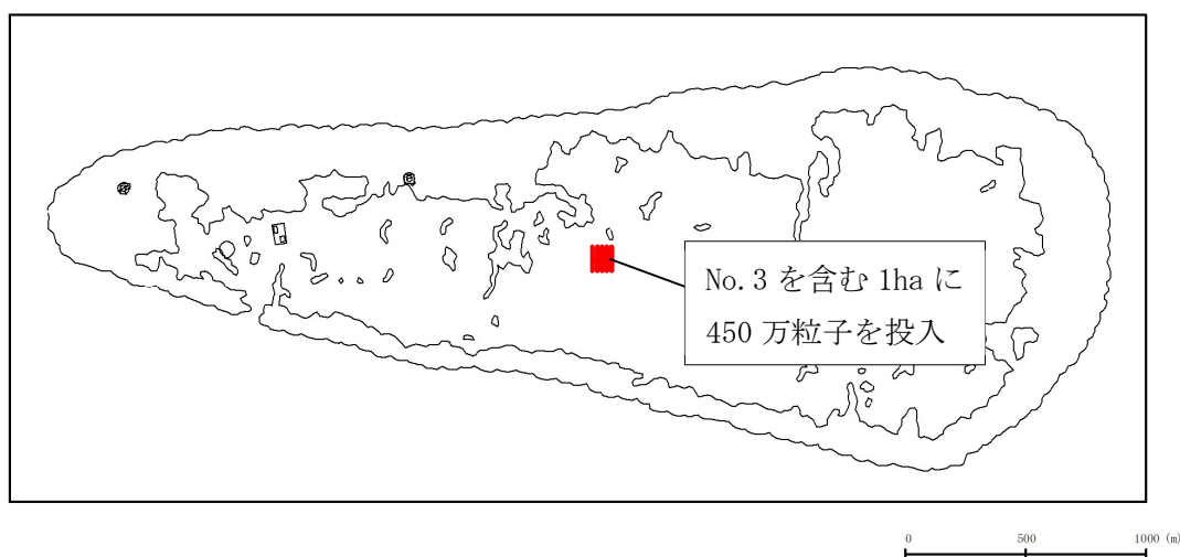
図-Ⅲ.2.2.15 粒子投入箇所
