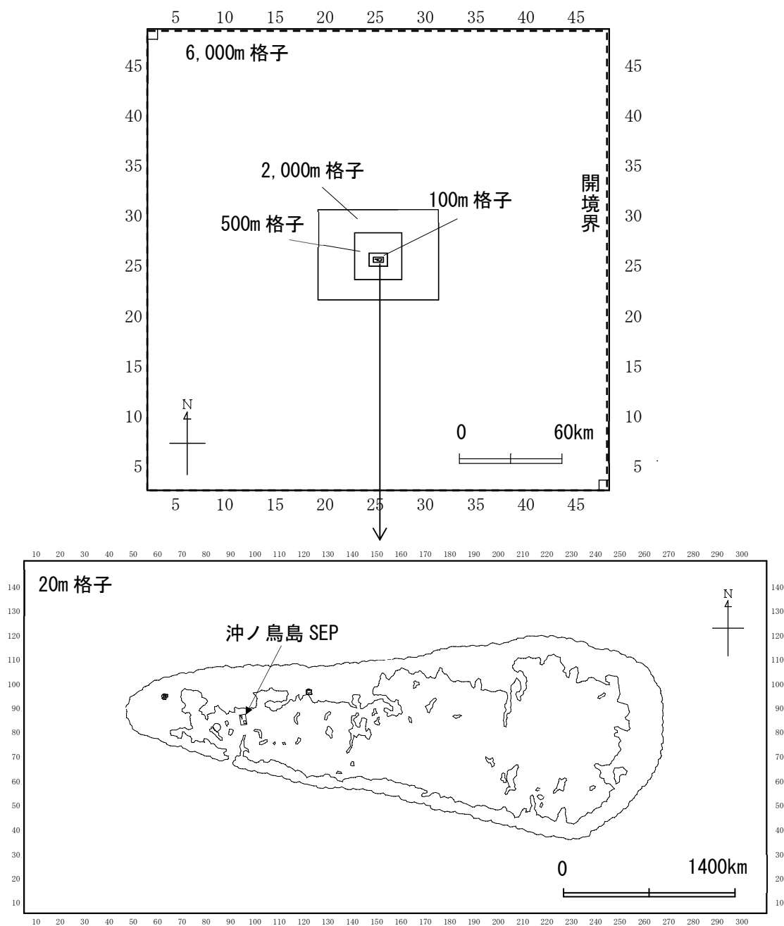
図-Ⅲ. 2. 2. 1 シミュレーションの計算範囲
