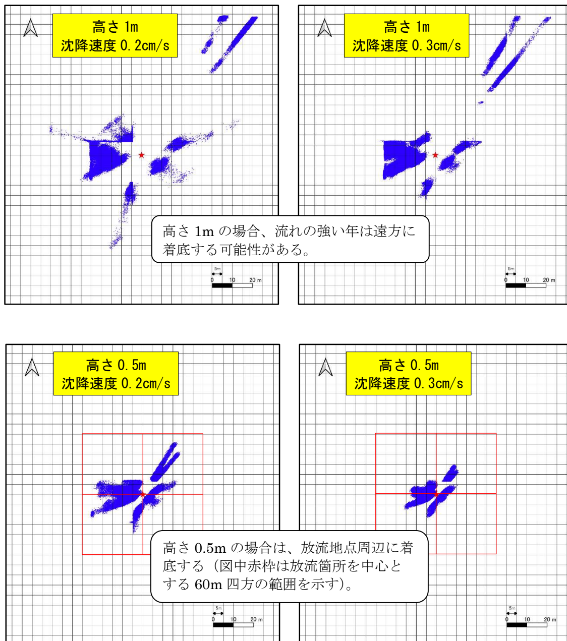
図-Ⅲ. 2. 2. 14 21年分の粒子着底位置
