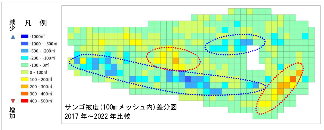
図-Ⅲ.2.1.3 サンゴ被度差分図 (上図：2017年~2022年比較)
