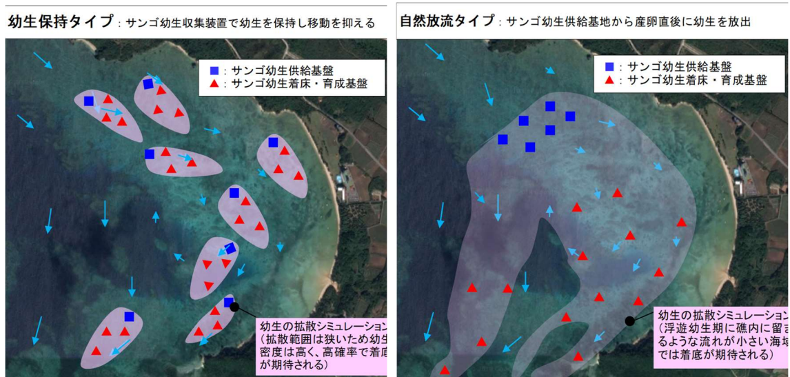
図-Ⅲ.2.1.1 サンゴ浮遊幼生の面的拡散イメージ
