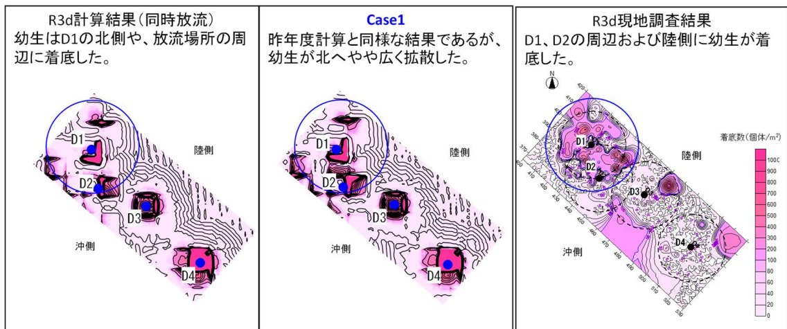
図-Ⅲ. 2. 1. 2 R3 年度の再現計算検証結果①（断続移動式放流）
