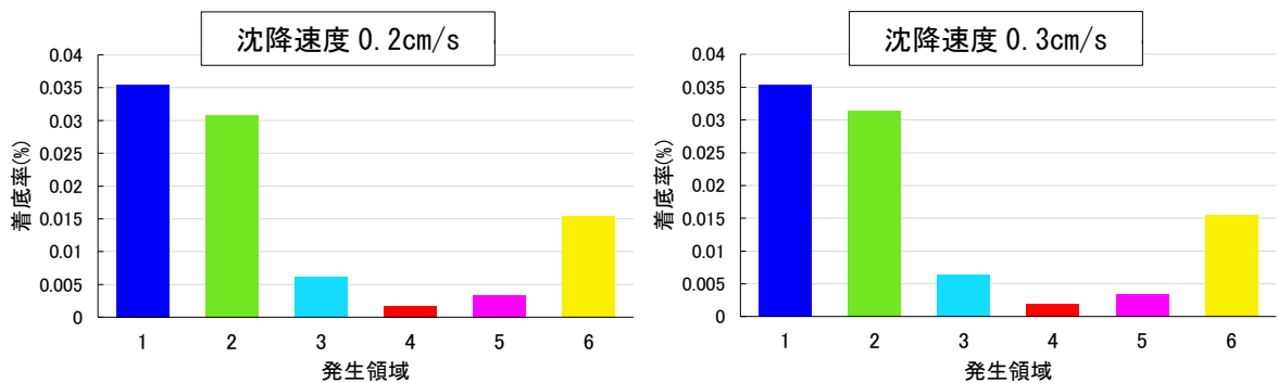
図-III.2.2.11 検討 2 の領域毎の着底率 (21 年平均 ※2013 年を除外)
