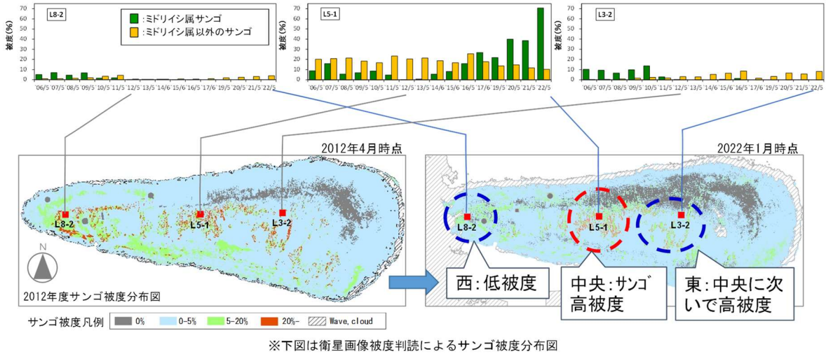
図-Ⅲ. 2. 1. 4 衛星画像被度判読によるサンゴ被度分布
