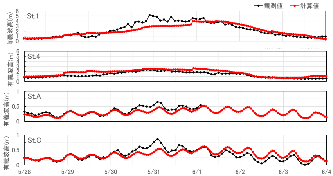
図-Ⅲ. 2. 2. 5 波浪モデルの再現性検証の比較（再現ケース②）
