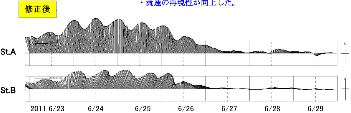
図-Ⅲ. 2. 2. 4 流動モデルの再現性検証の比較（再現ケース①）
