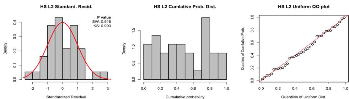
補足図 1-1a. HS 型再生産関係における（左）標準化残差のヒストグラムと正規性テスト結果、（中央）残差の累積確率密度のヒストグラム、（右）一様分布を仮定した QQ プロット
