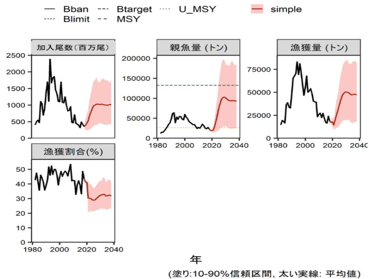
補足図 4-2. シナリオ②の MSE 将来予測（真の再生産関係が BH 型と仮定し、RI 型の漁獲管理規則案を用いた場合） 太実線は平均値、網掛けはシミュレーション結果の 80%が含まれる 80%予測区間。親魚量の図の破線は BH 型の管理基準値案（緑：目標管理基準値案、黄：限界管理基準値案）。2019 年と 2020 年の漁獲量は予測される資源量と F_{current} により仮定し、2021 年以降の漁獲は漁獲管理規則案に基づく（図 5）。安全係数 \beta には 0.8 を用いた。
