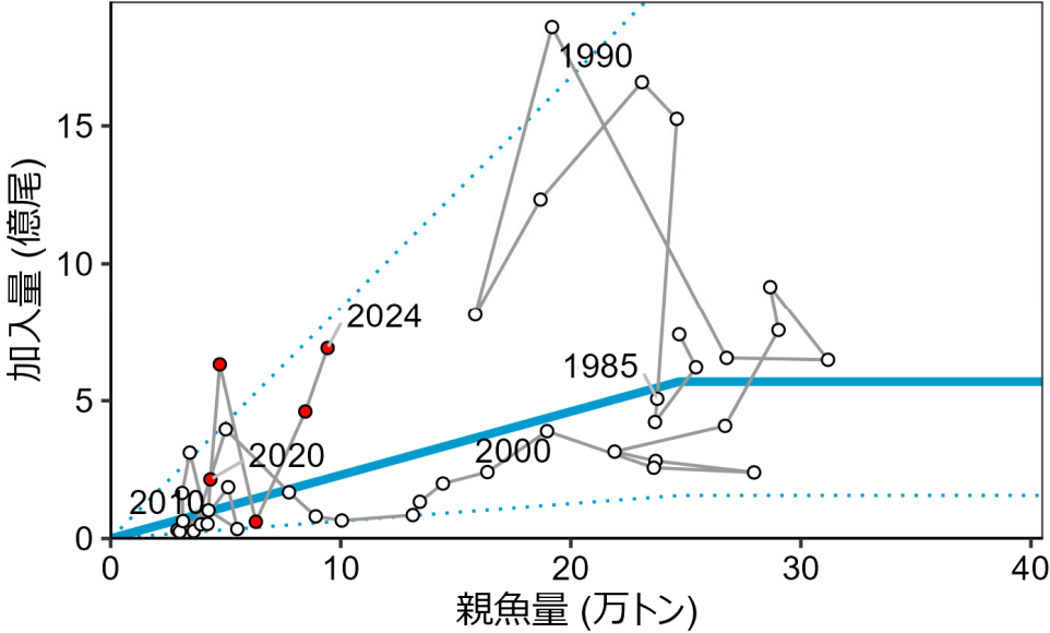
図8 再生産関係
