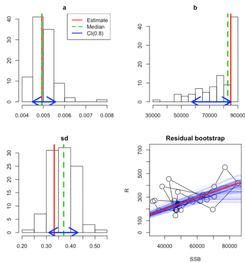
補足図 1-6. HS-L1 のパラメータ推定値に対するブートストラップ検定結果
