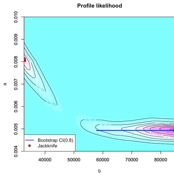
補足図 1-10. HS-L1 のパラメータ推定値のプロファイル尤度
