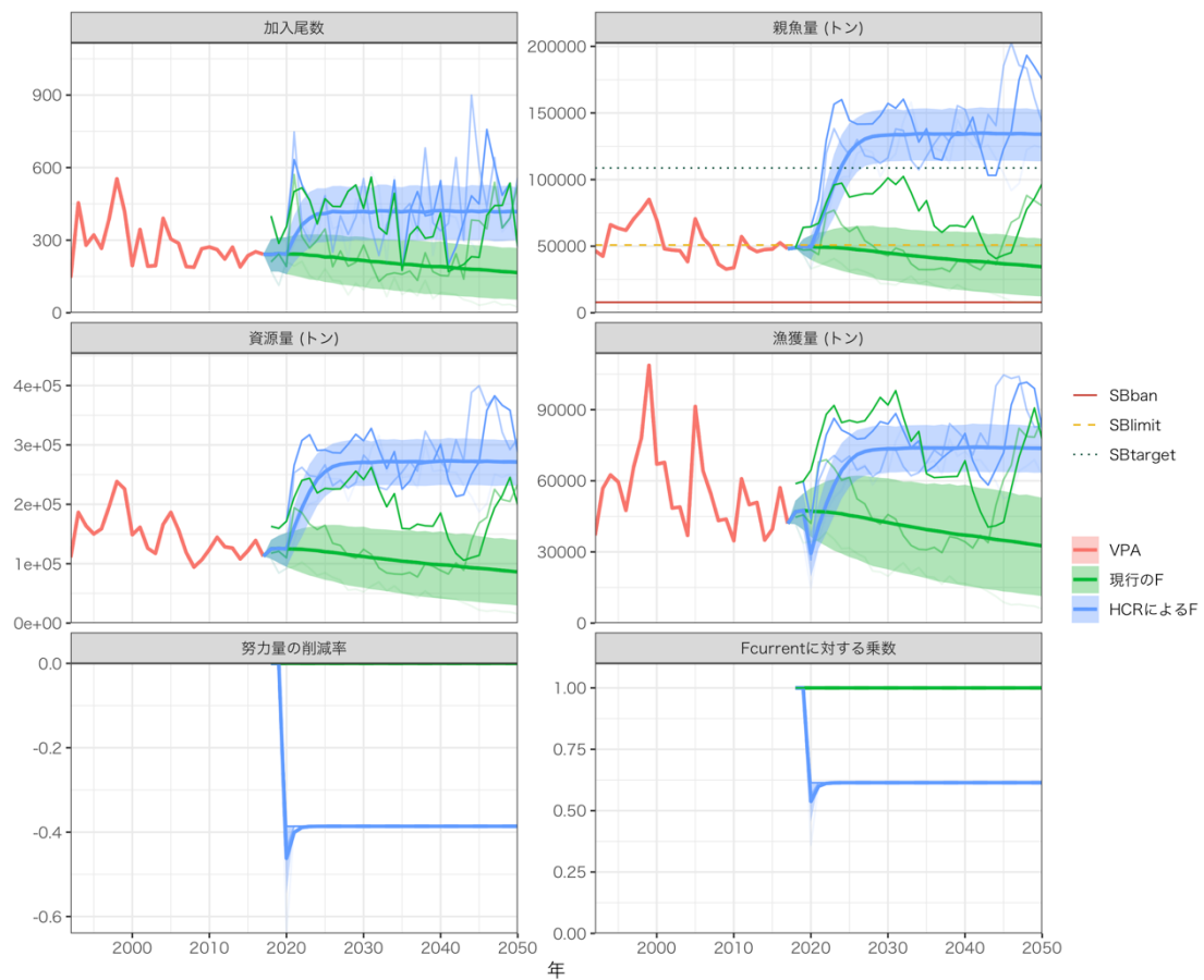
図 6. 漁獲管理規則による将来予測の平均値（実線）と 80%信頼区間
