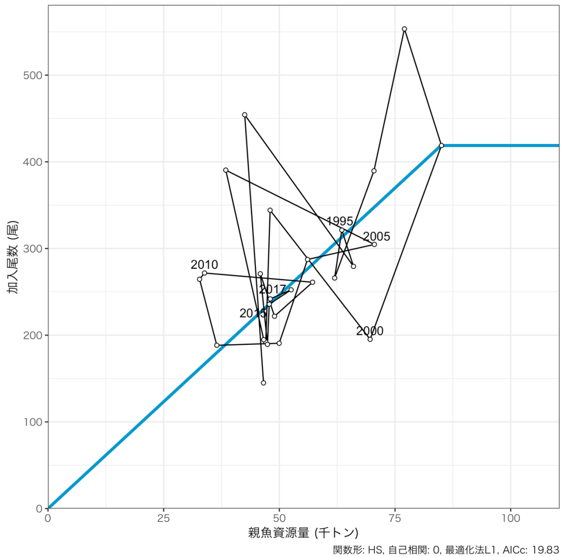
図 1. 再生産関係
