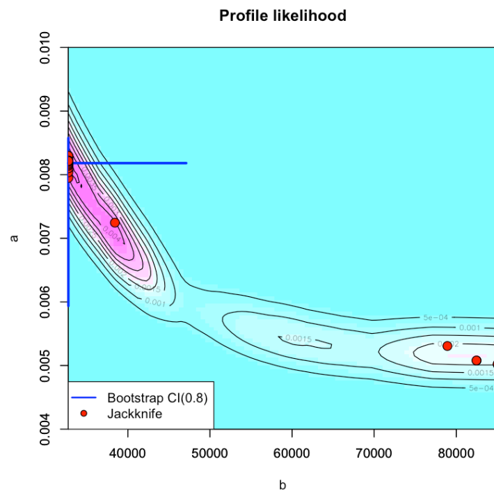
補足図 1-11. HS-L2 のパラメータ推定値のプロファイル尤度
