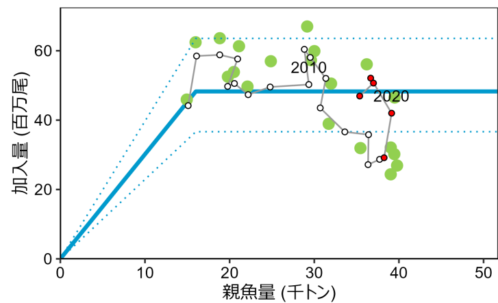
図6 再生産関係
