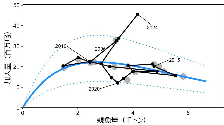
図4 再生産関係
