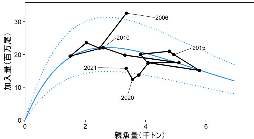
図4 再生産関係
