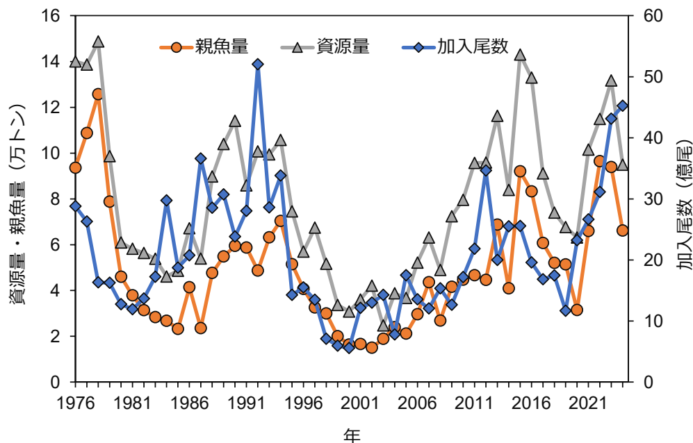
図4 資源量・親魚量・加入量
