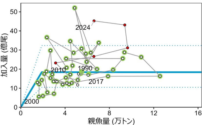
図6 再生産関係
